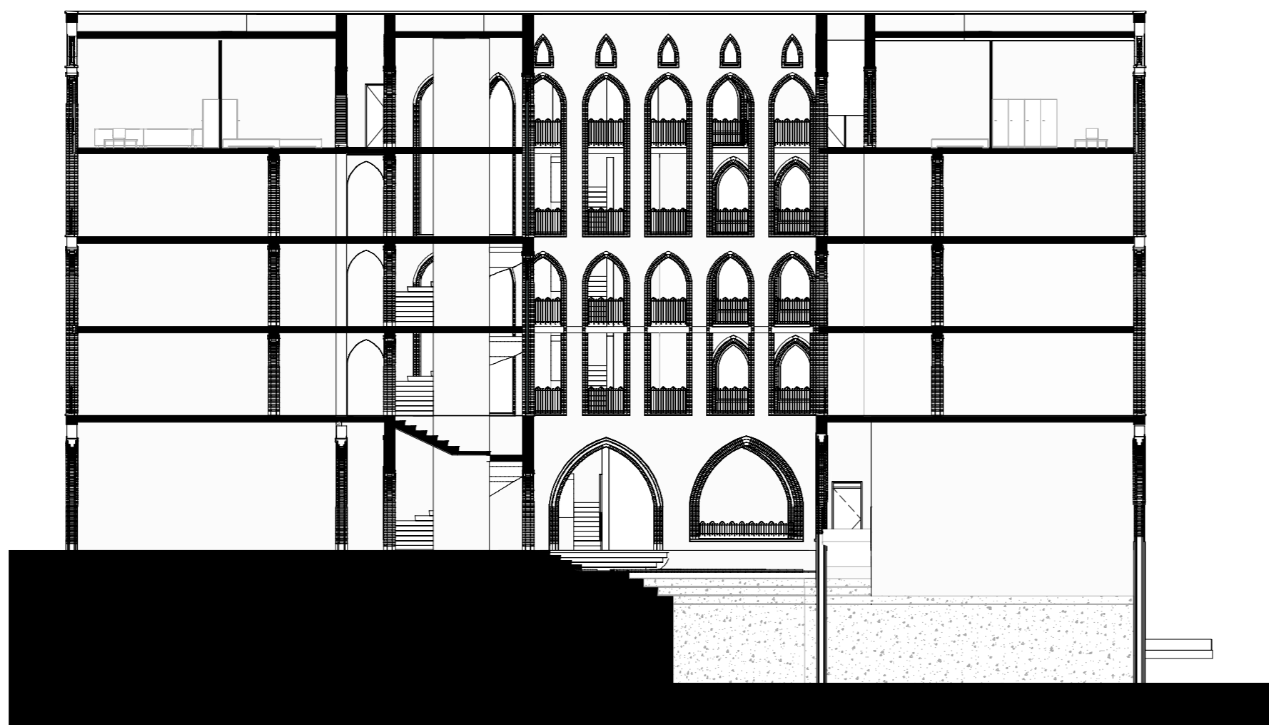
Doorsnede
