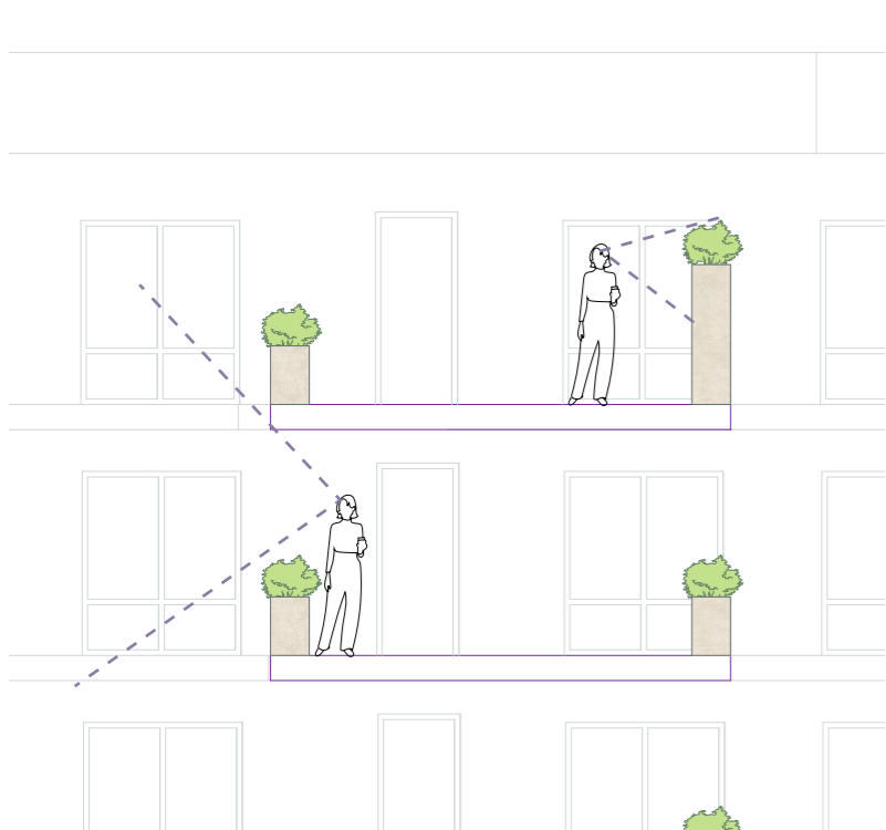
Dwarsdoorsnede 1:100
