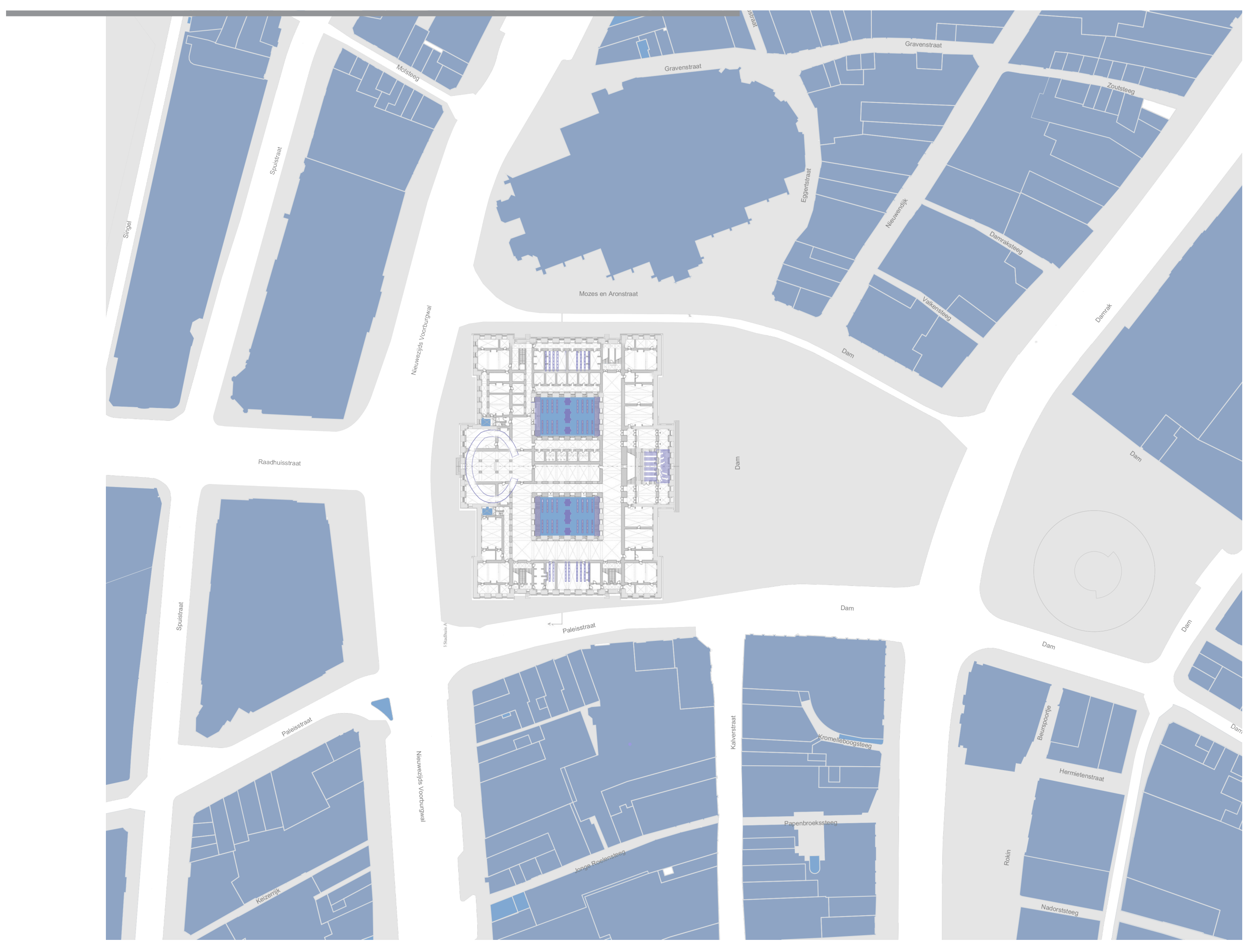
Situatie 1:1000
