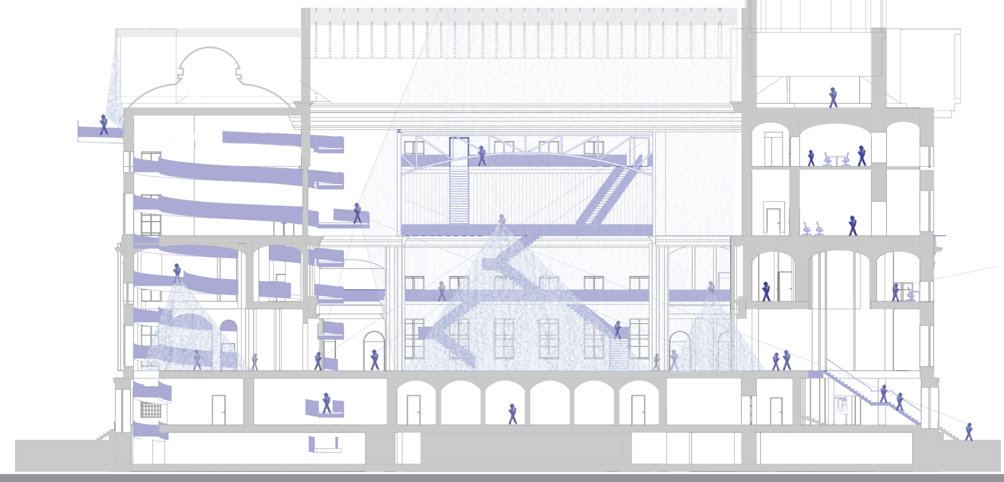
Doorsnede B nieuwe situatie 1:300
