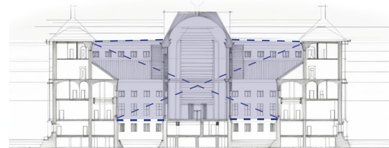
Schematische weergave nieuwe atrium doorsnede A
