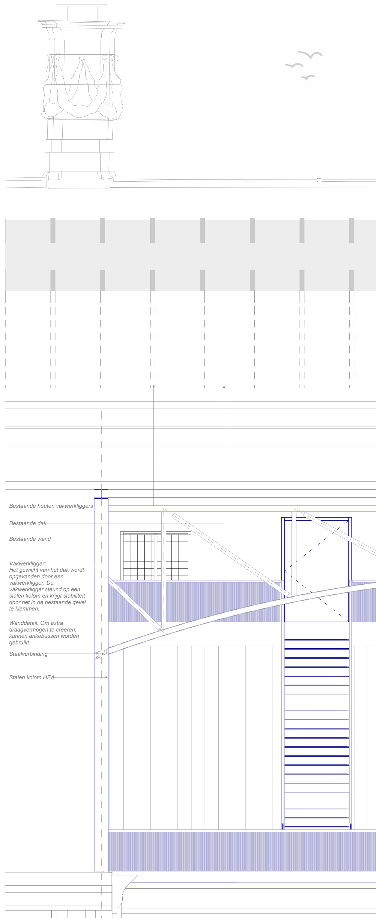
Fragment vakwerklijger 1:50
