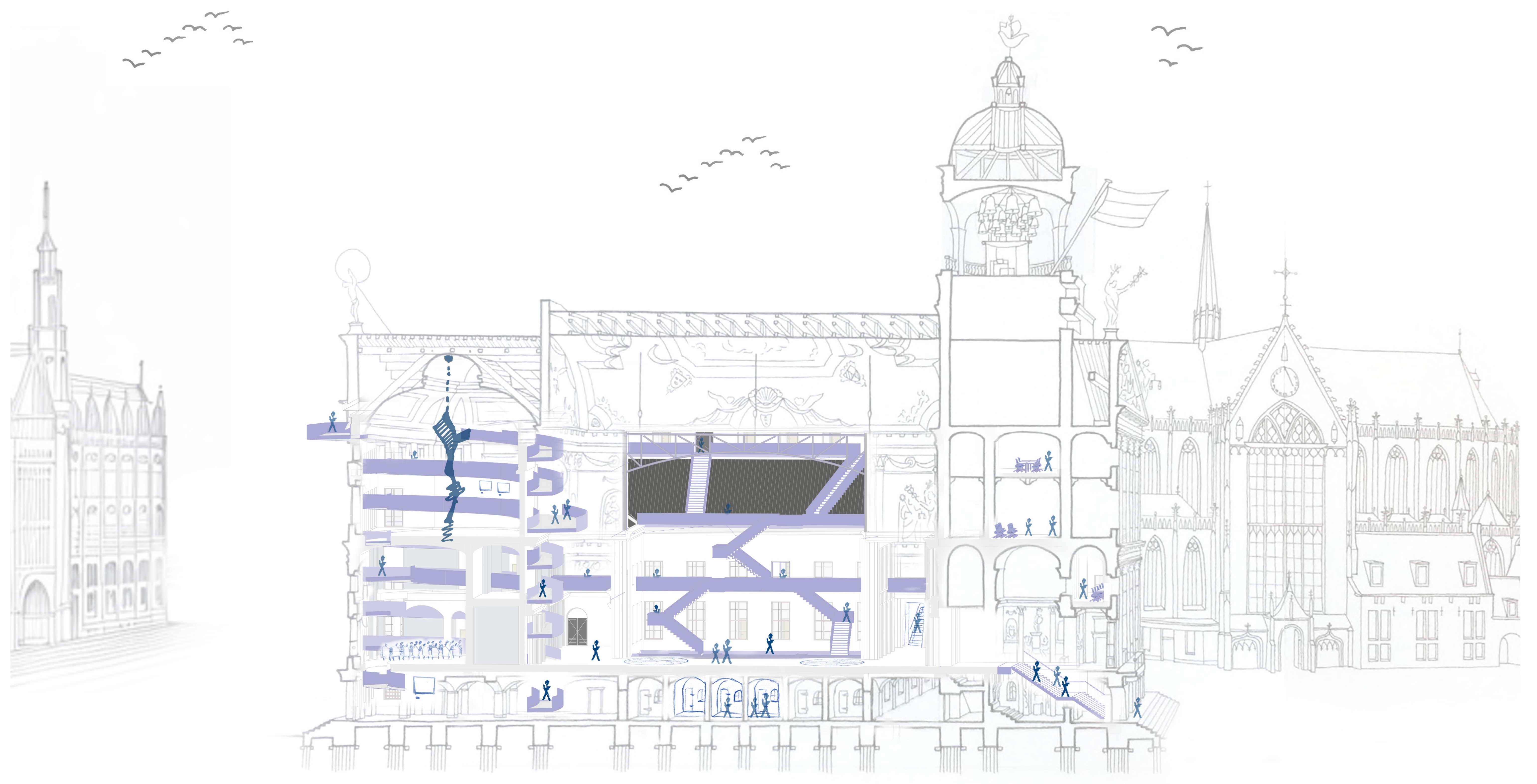
Doorsnede A nieuwe situatie 1:300
