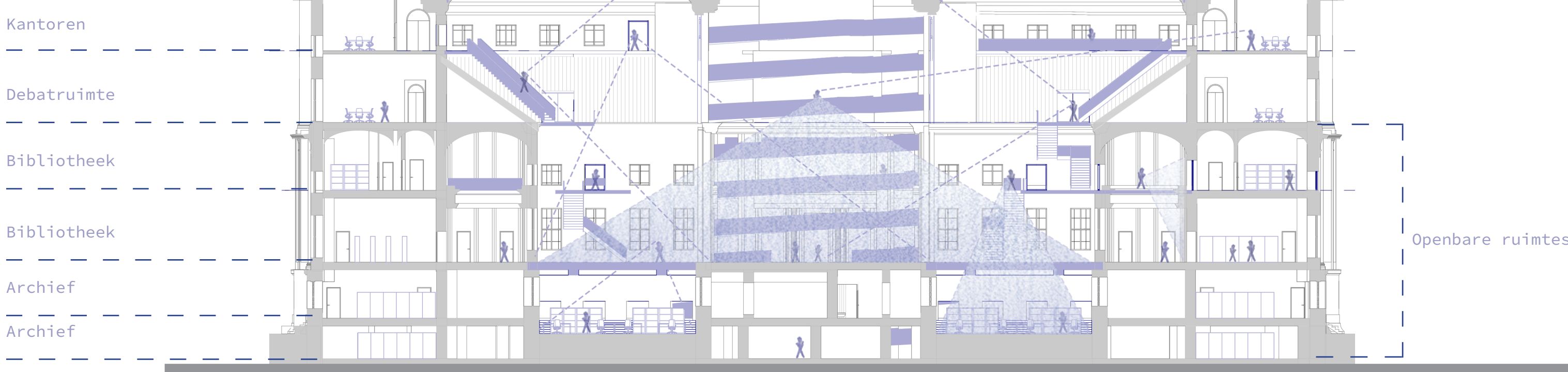
Doorsnede A nieuwe situatie 1:300
