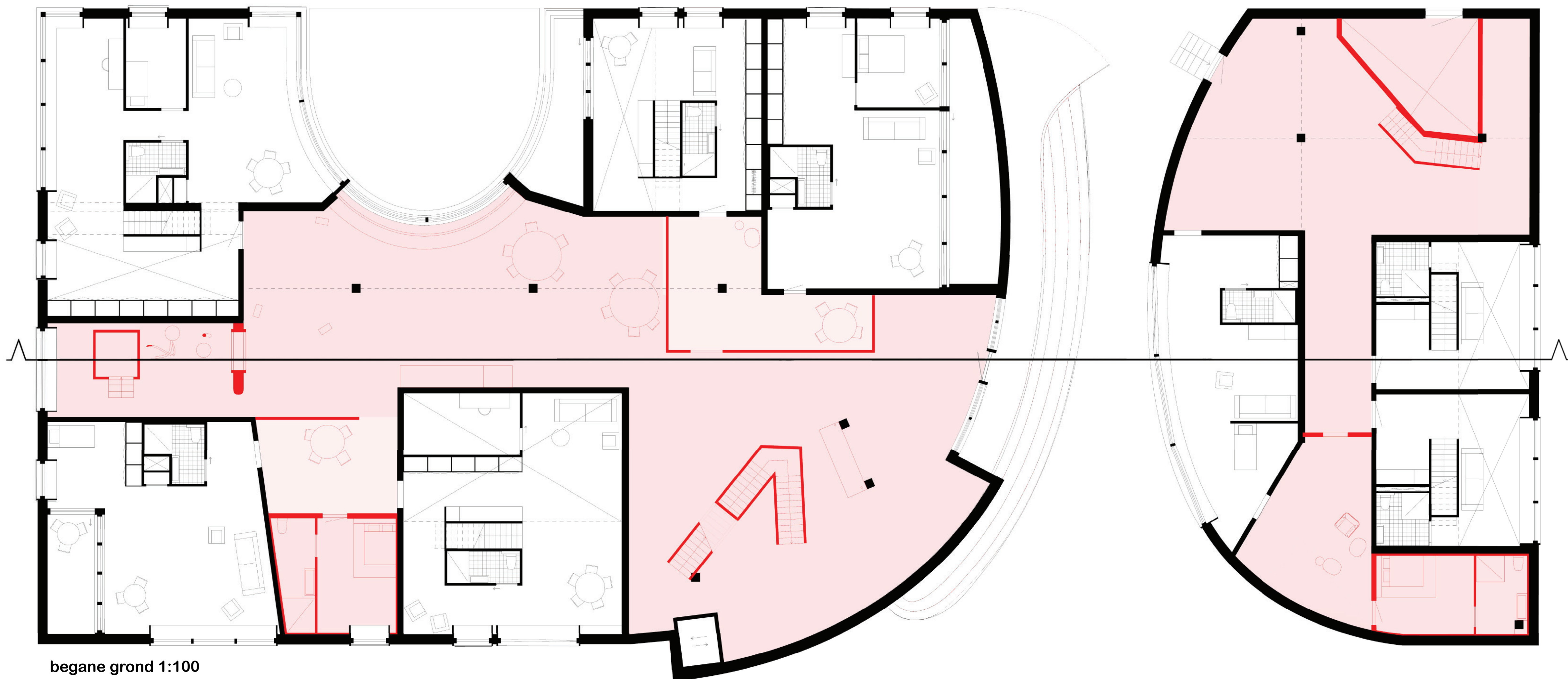
begane grond 1:100
