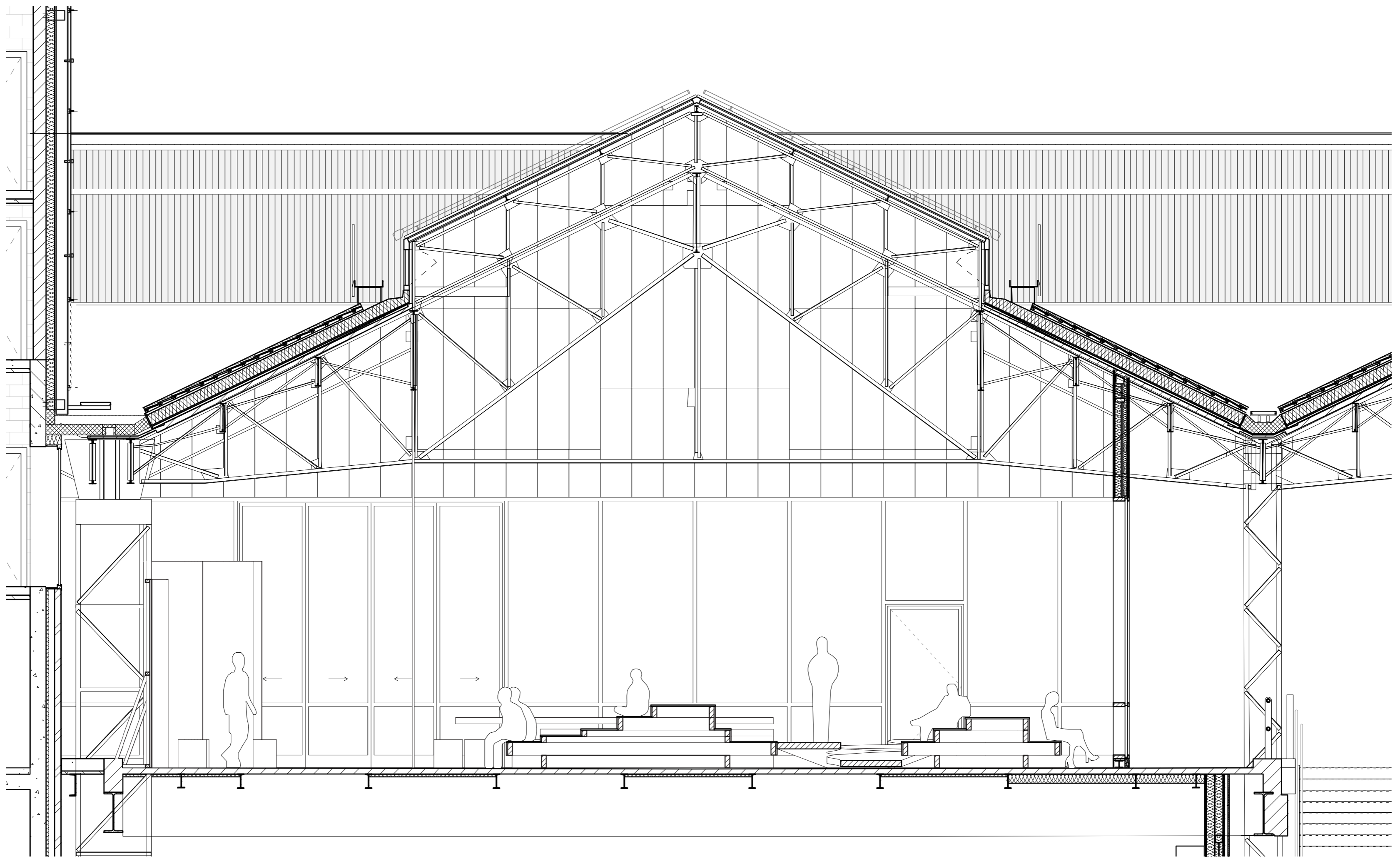
Doorsnede 1:50
