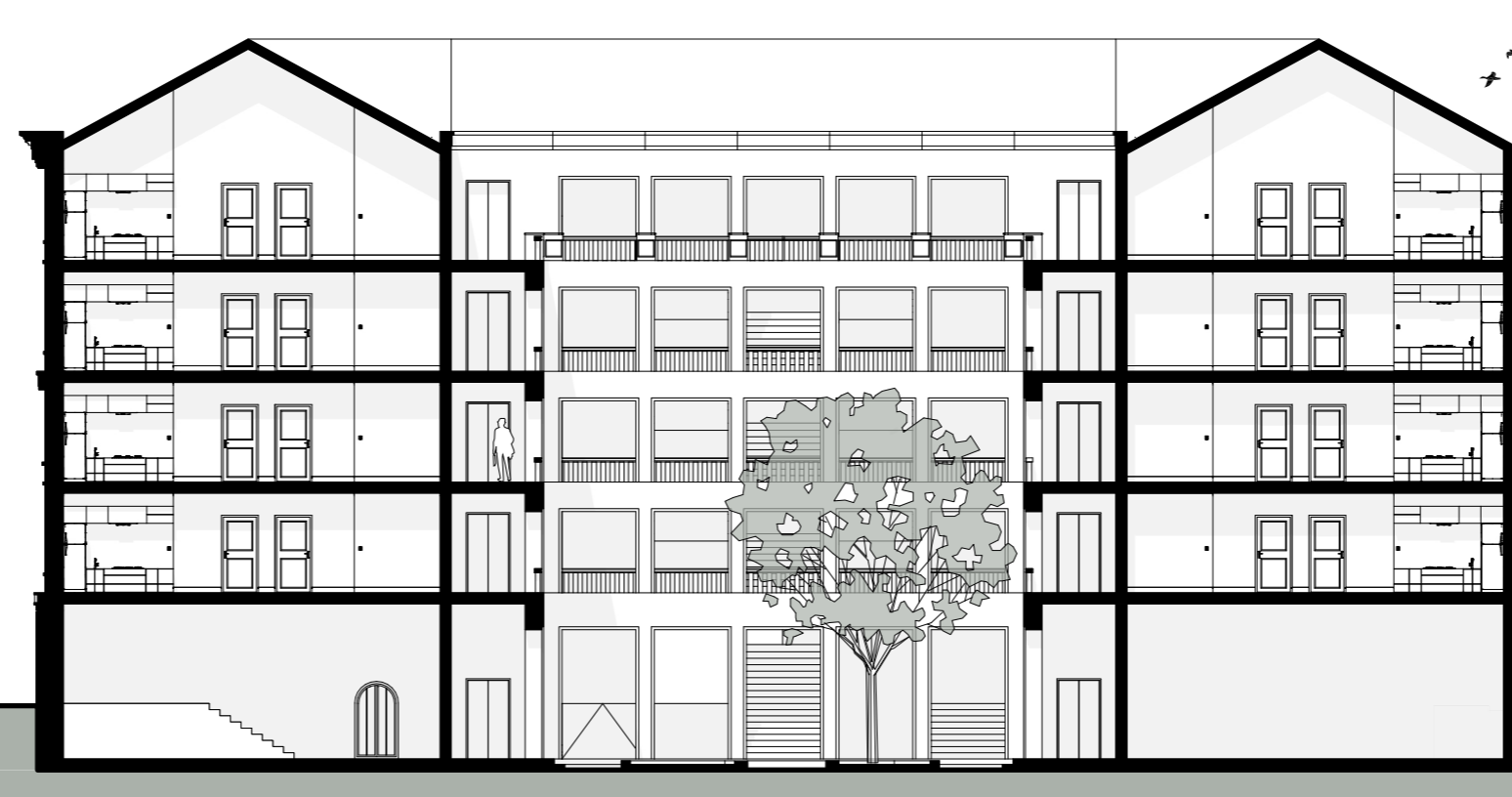
DOORSNEDE B-B 1:200
