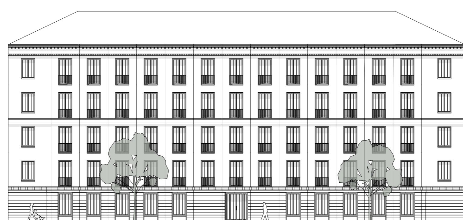
LINKERZIJGEVEL 1:200
