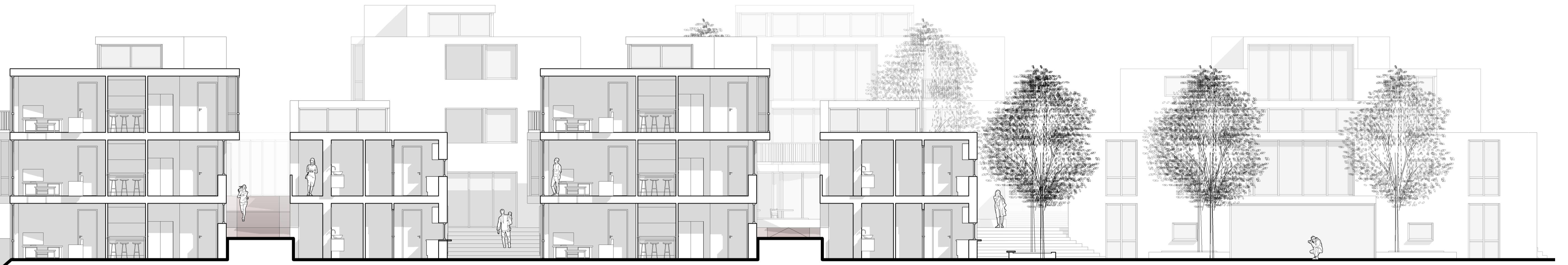
DOORSNEDE OVER DE WONINGEN 1:100
