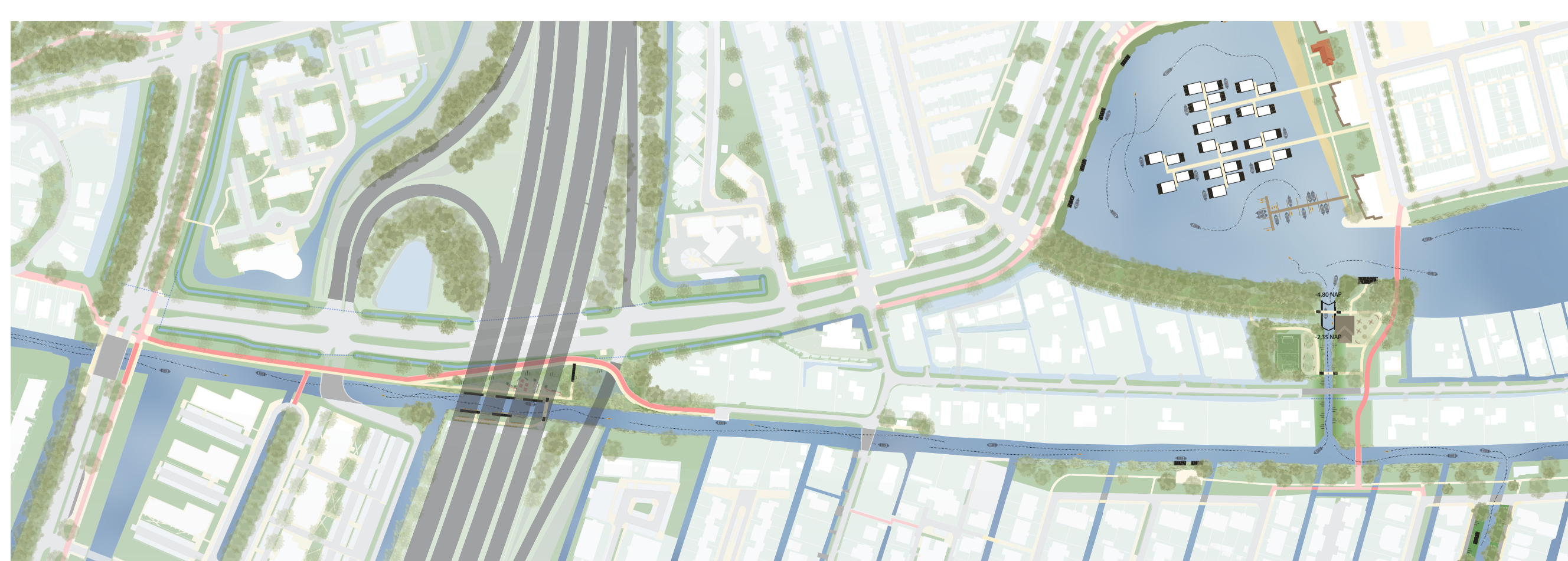
Plattegrond op de plek waar de A16 en de Ringvaart elkaar kruisen en waar de Ringvaart verbonden wordt met de Ringvaartplas.
