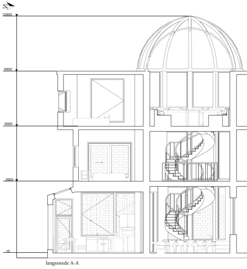
langsnede A-A
