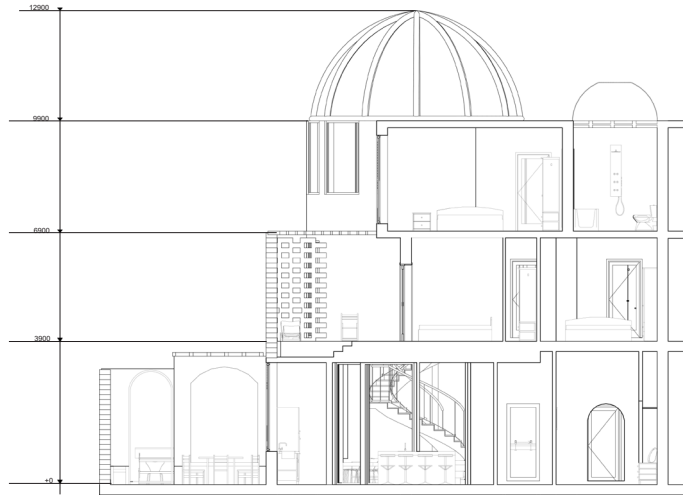
langsnede B-B
