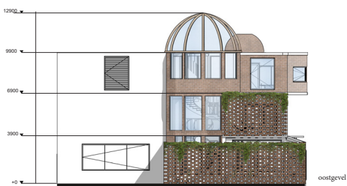
oostgevel
