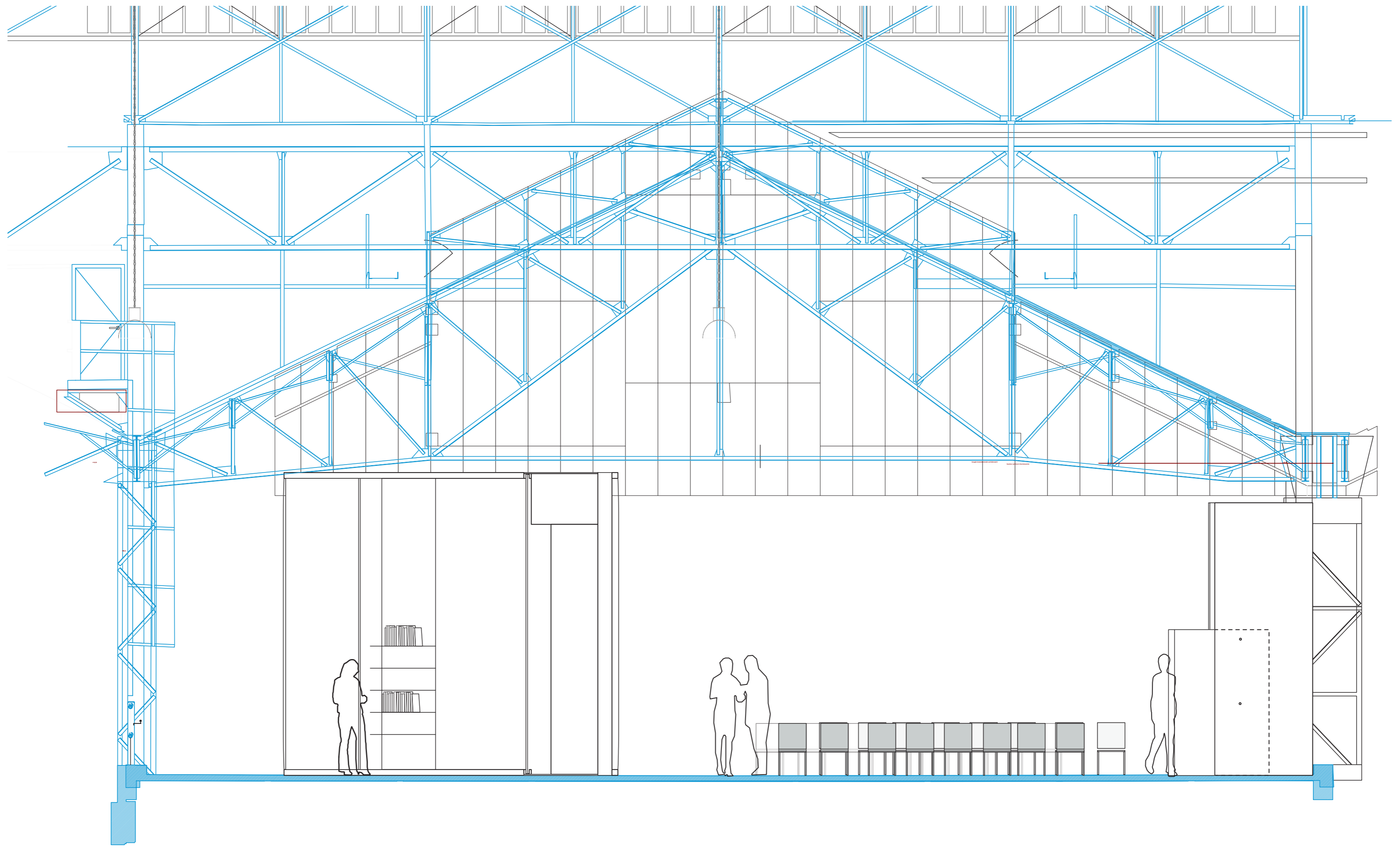
Doorsnede 1:50
