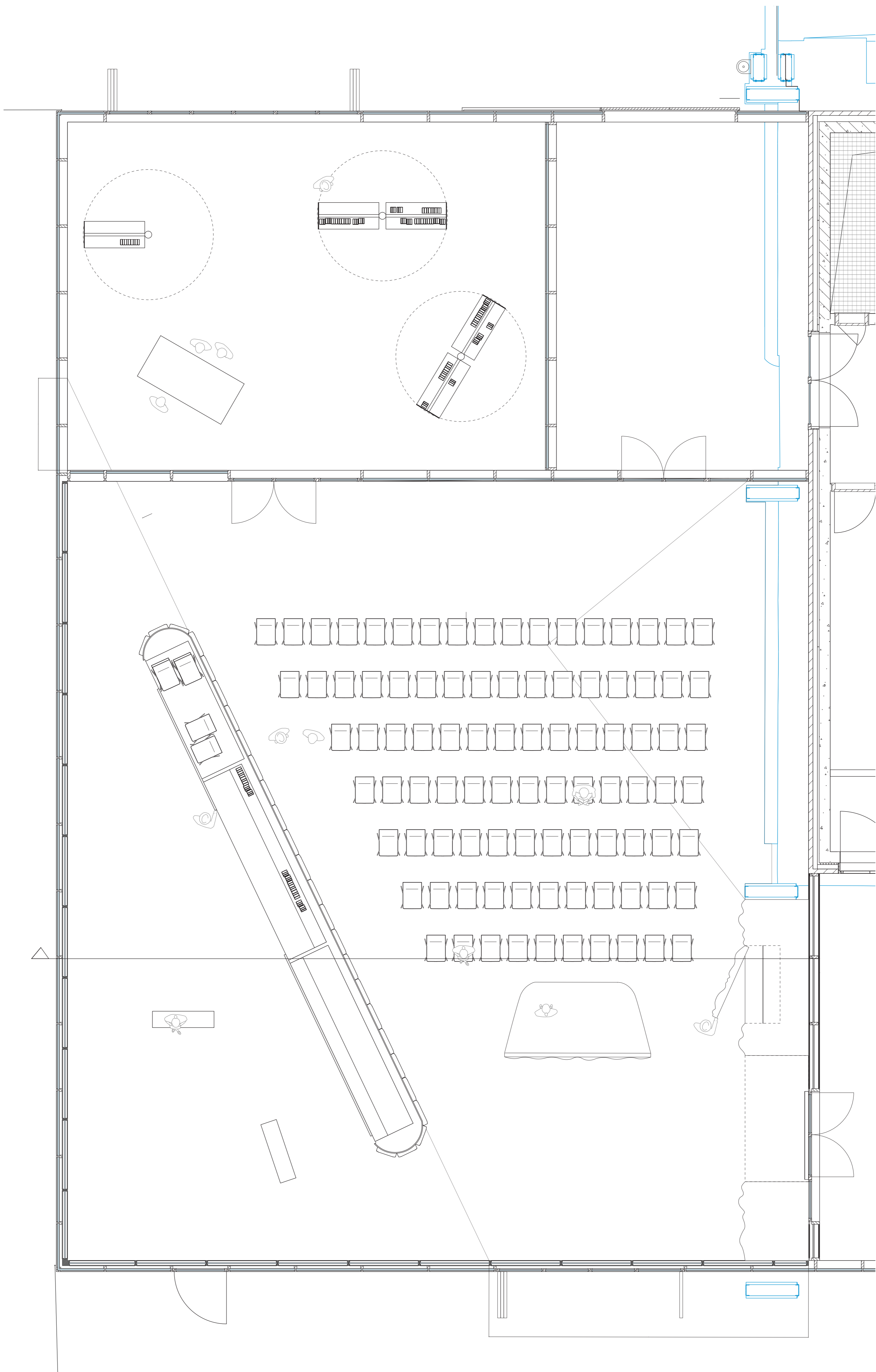
Plattegrond 1:50
