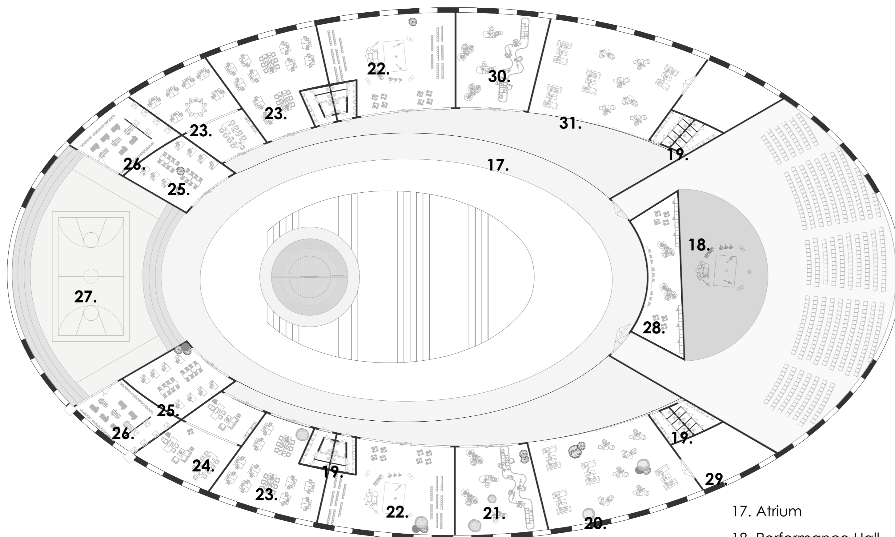
First floor Scale: 1:350
