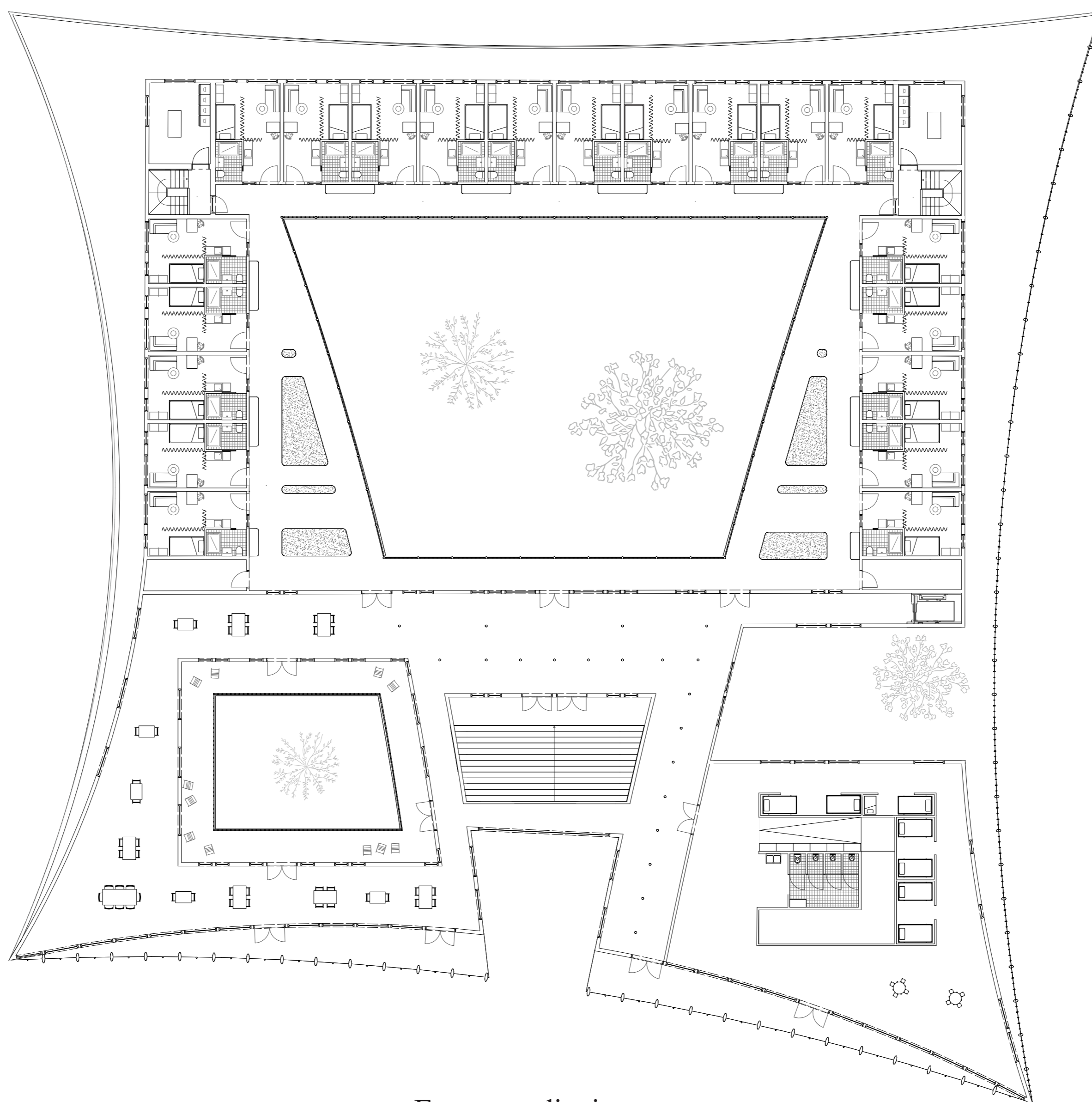
Eerste verdieping schaal 1:200
