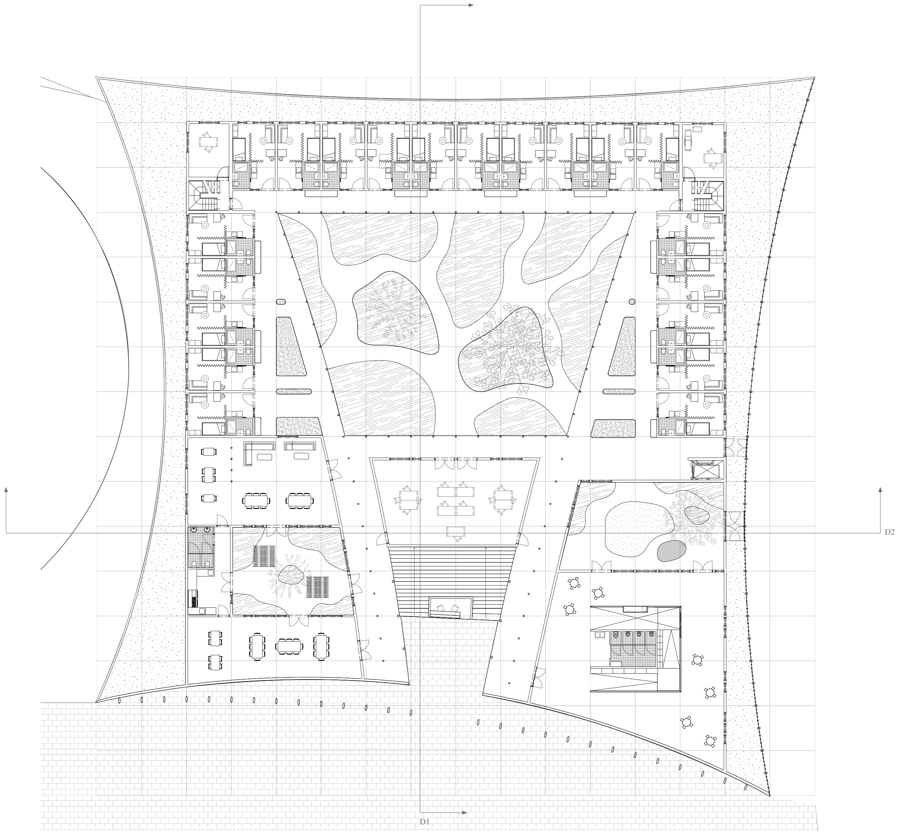
Begane grond schaal 1:200
