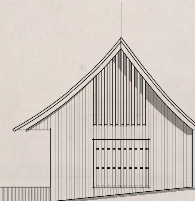
Noordgevel nieuw
