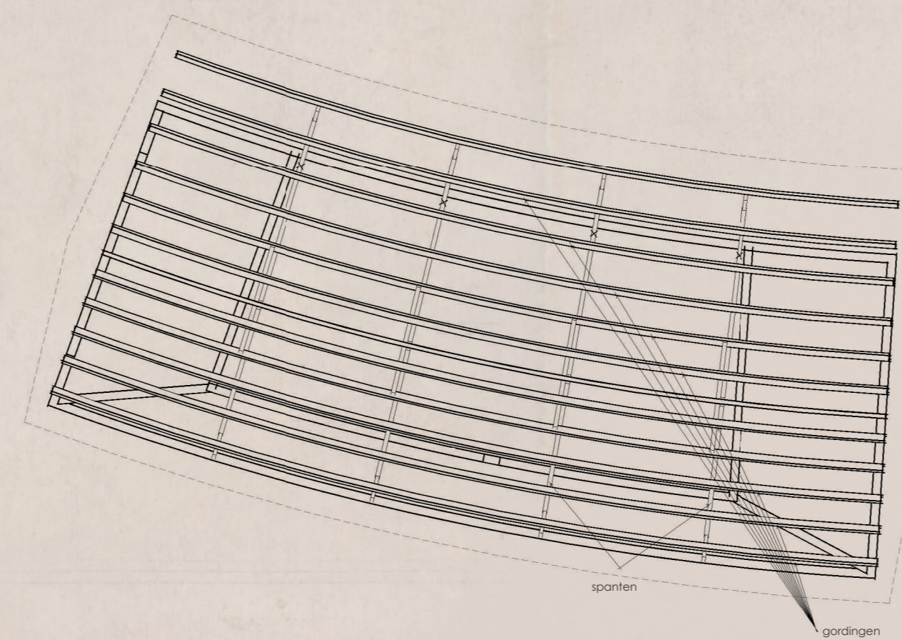
Kap constructie
