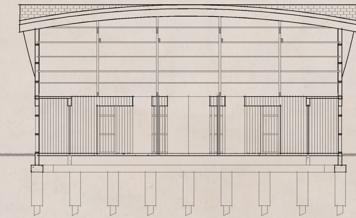
Doorsnede B nieuw
