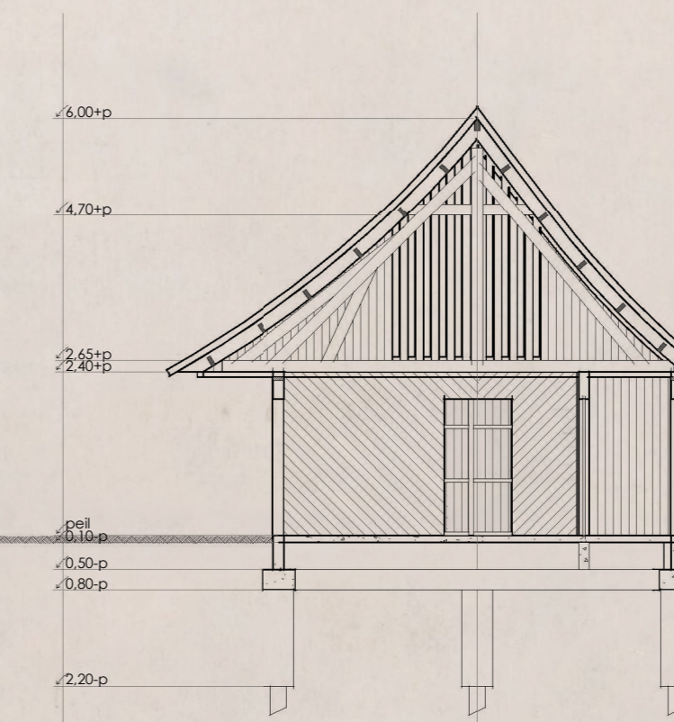
Doorsnede A nieuw
