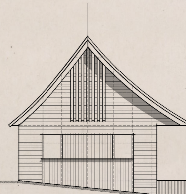
Zuidgevel bestaand
