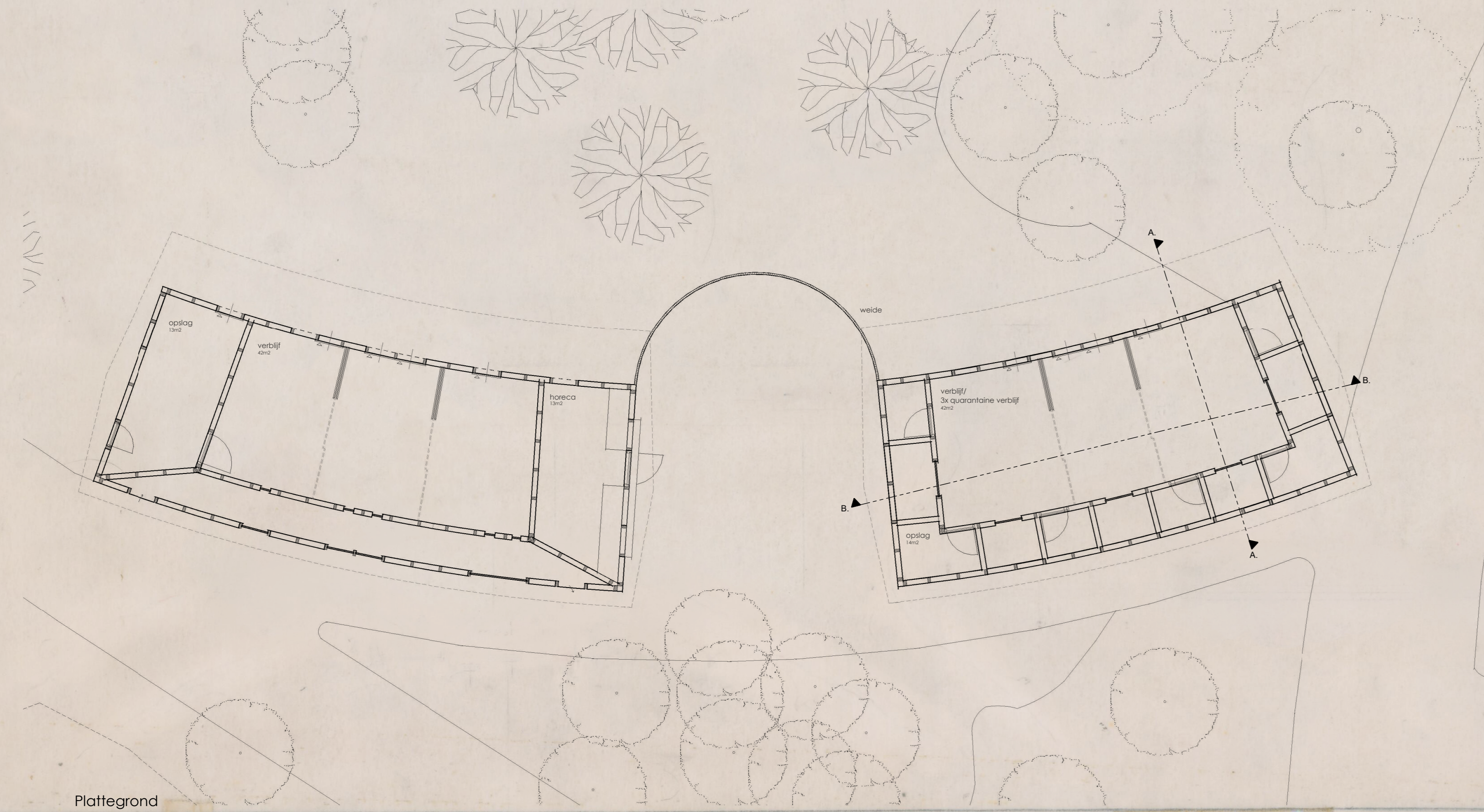
Plattegrond
