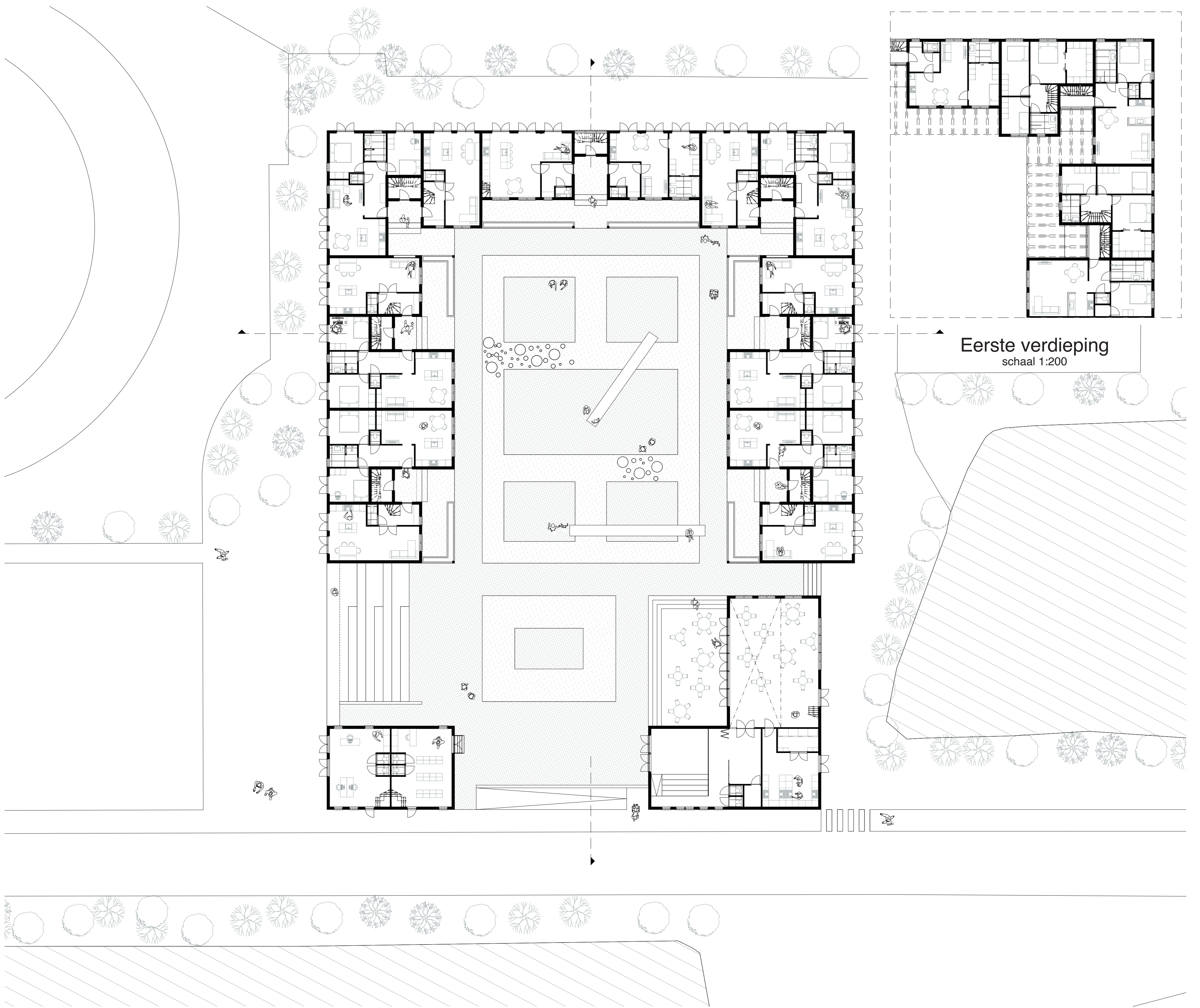
Begane grond schaal 1:200
