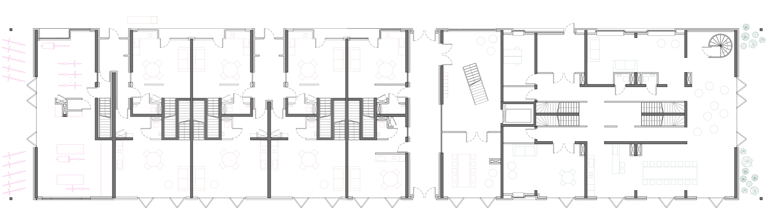
PLATTEGROND BEGANE GROND 1/200
