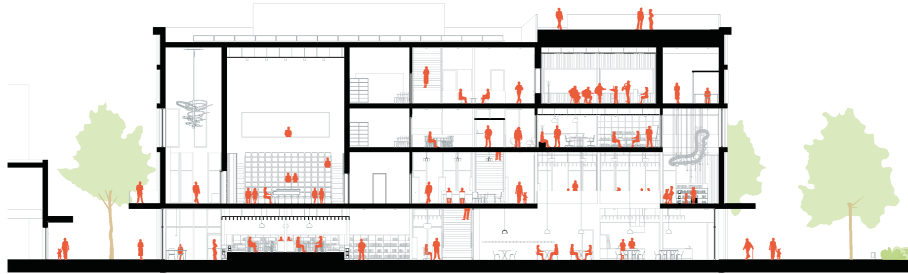
Doorsnede AA
