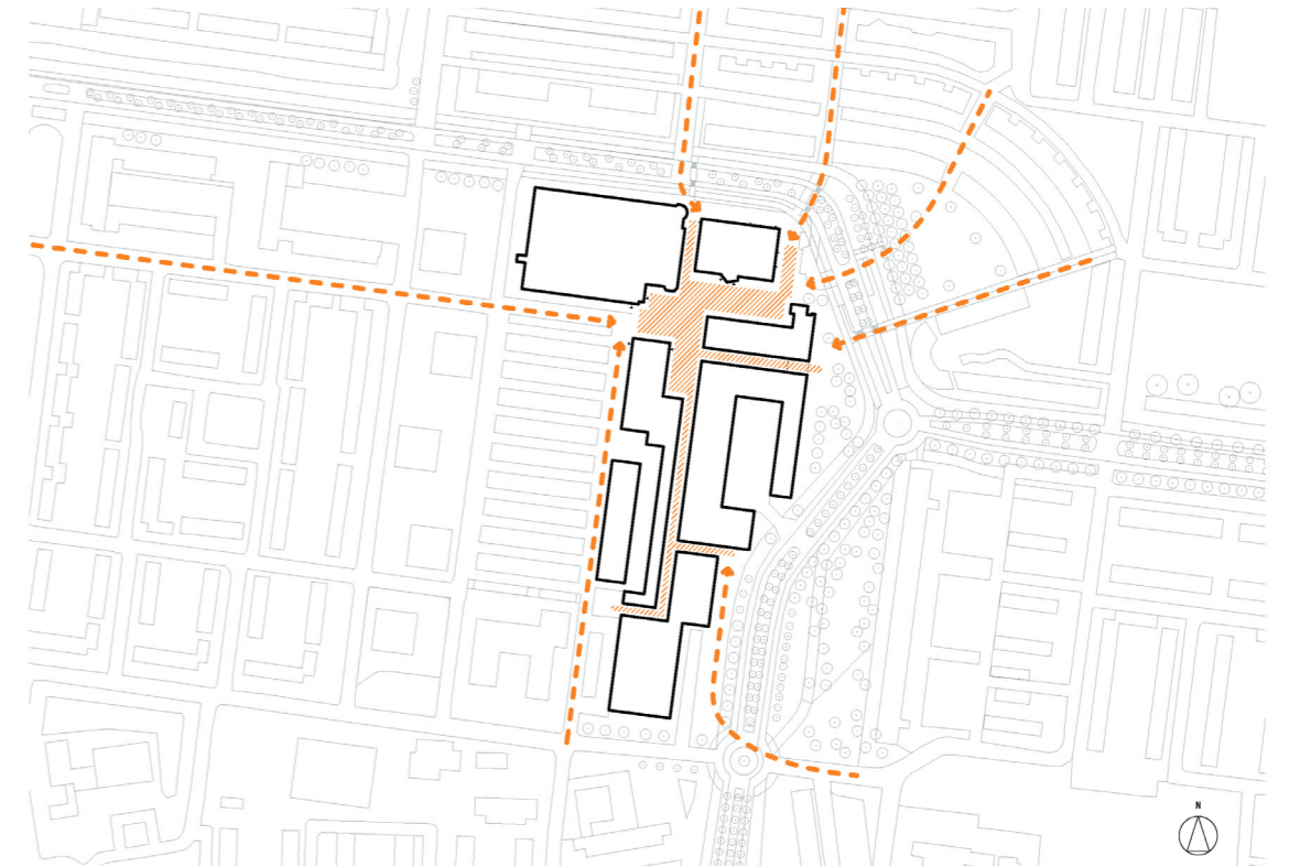
Beoogde situatie: het winkelcentrum terugbrengen naar een doorwaadbare plek zoals het vroeger was, dat beter aansluit op de wijk en de wijk een impuls geeft middels het nieuwe cultuurhuis.
