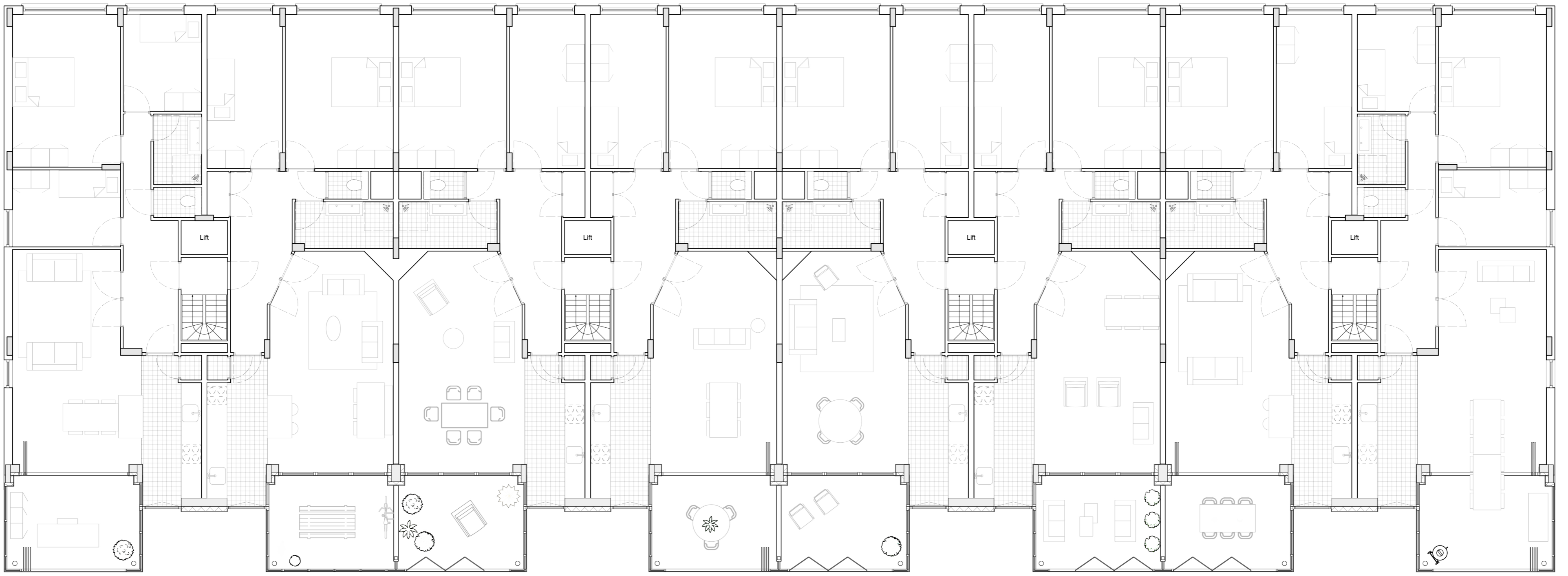
Verdieping nieuwe situatie 1.100
