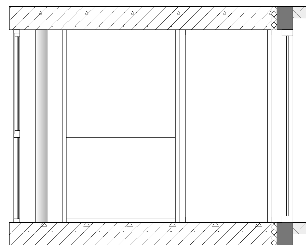
Verticale doorsnede 1.25
