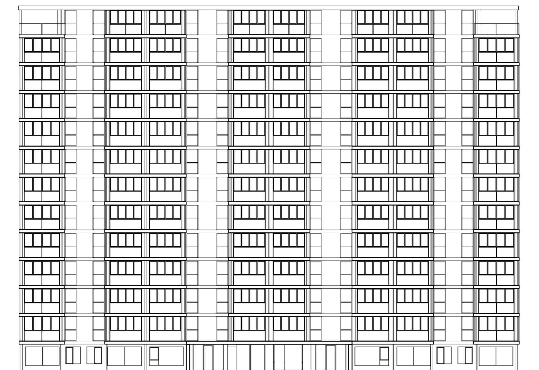
Voorgevel 1.200
