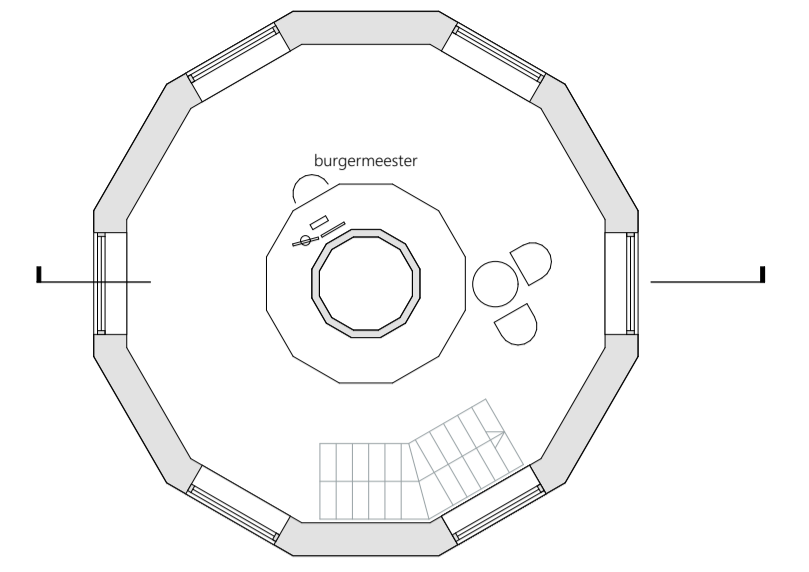
+4 1:100
