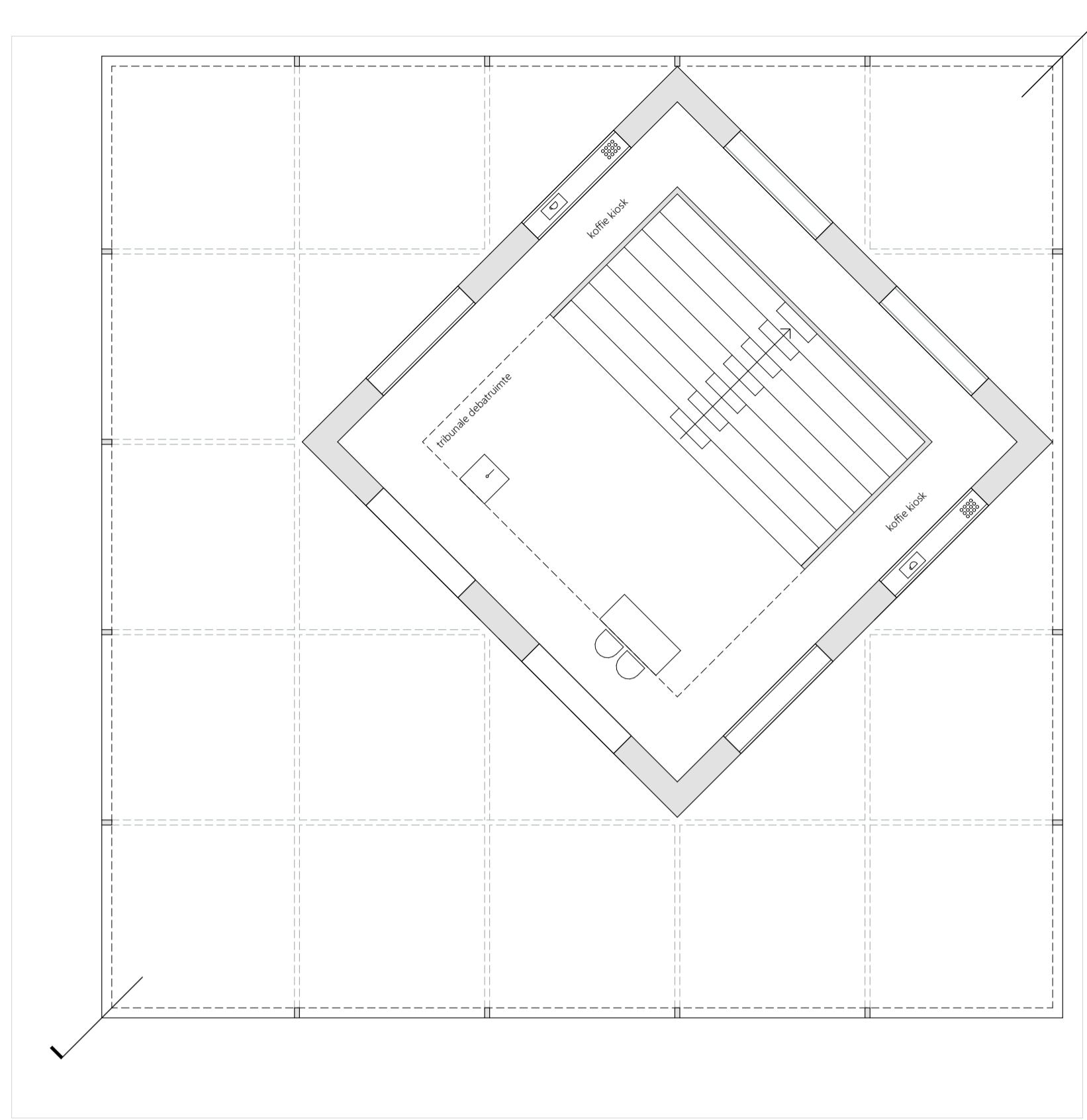
begane grond 1:100
