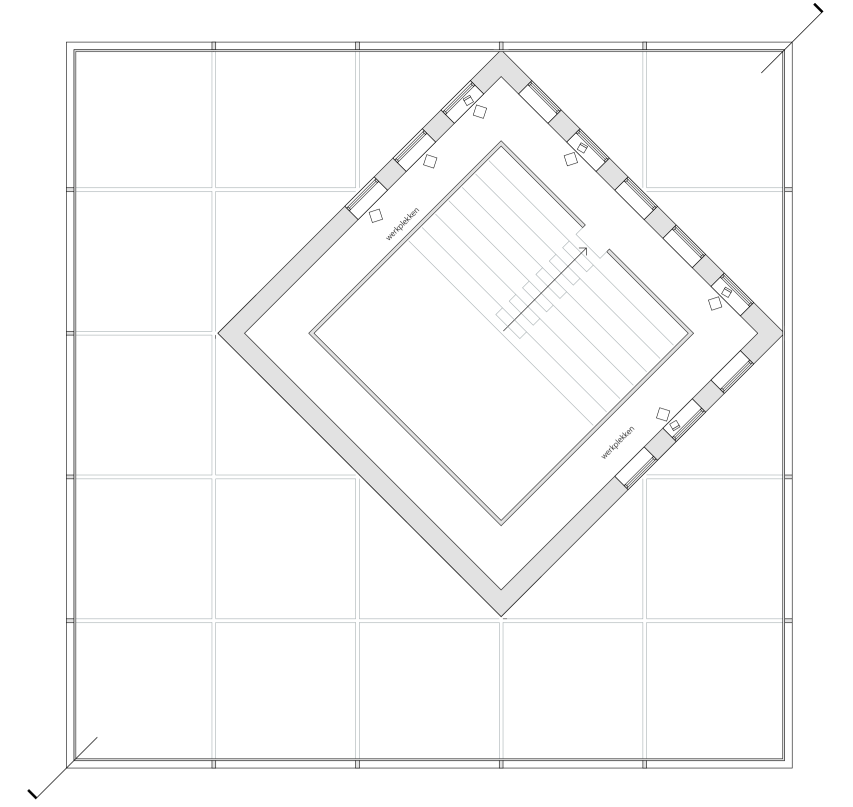
+1 1:100
