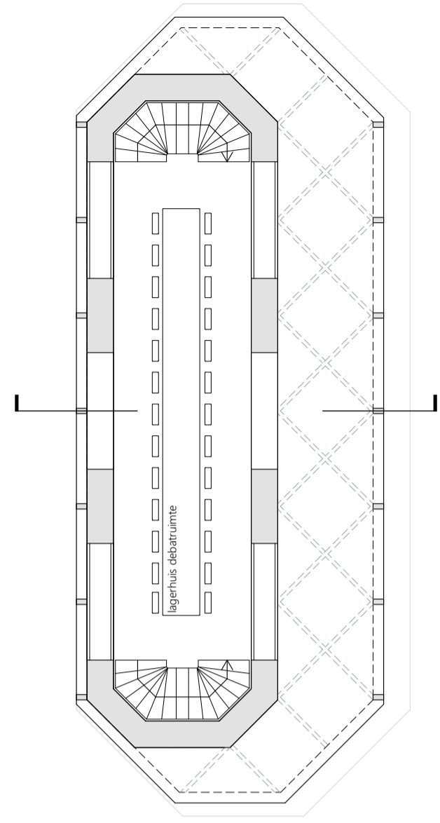
begane grond 1:100
