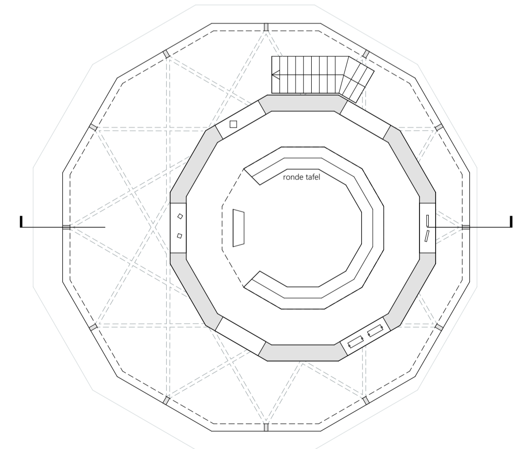
begane grond 1:100
