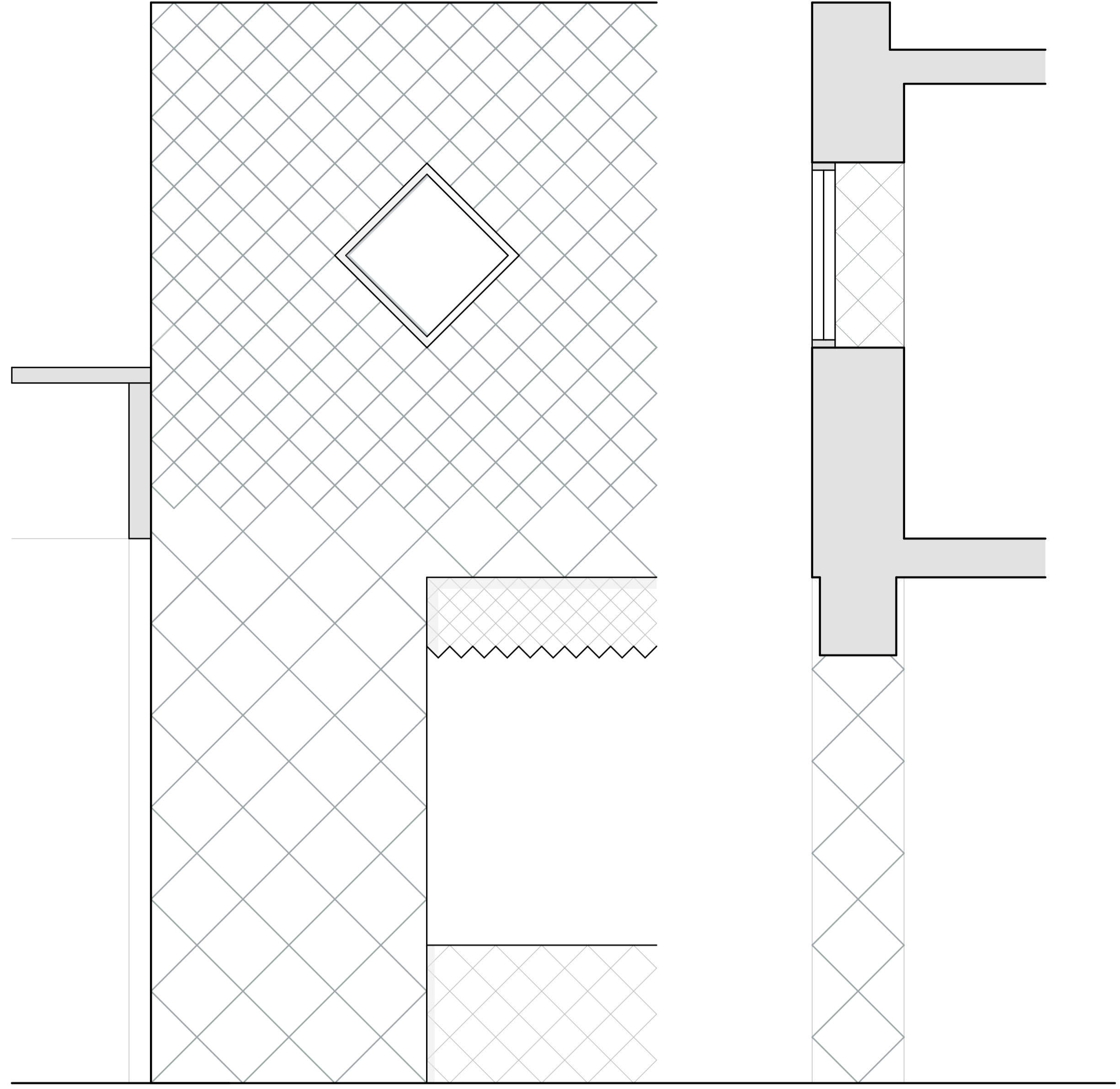
fragment tegelwerk 1:25
