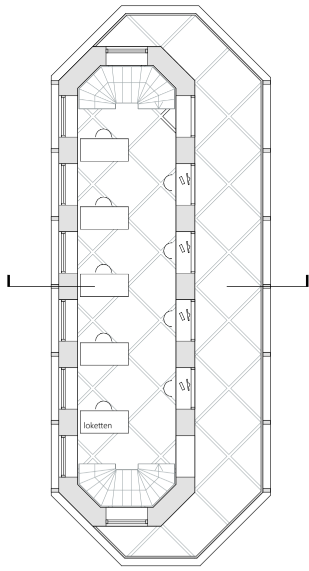
+1 1:100
