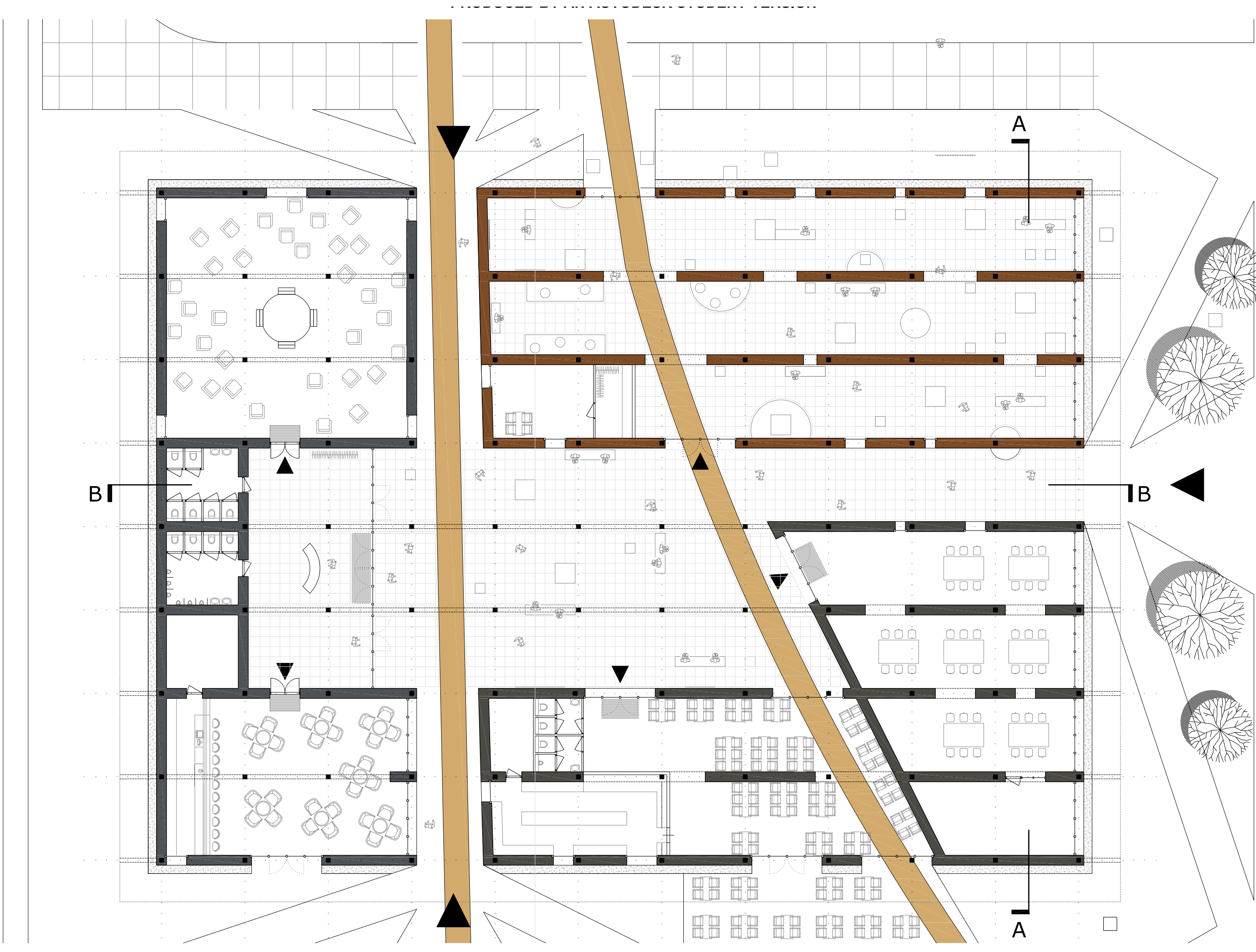
Floor plan 1 : 200
