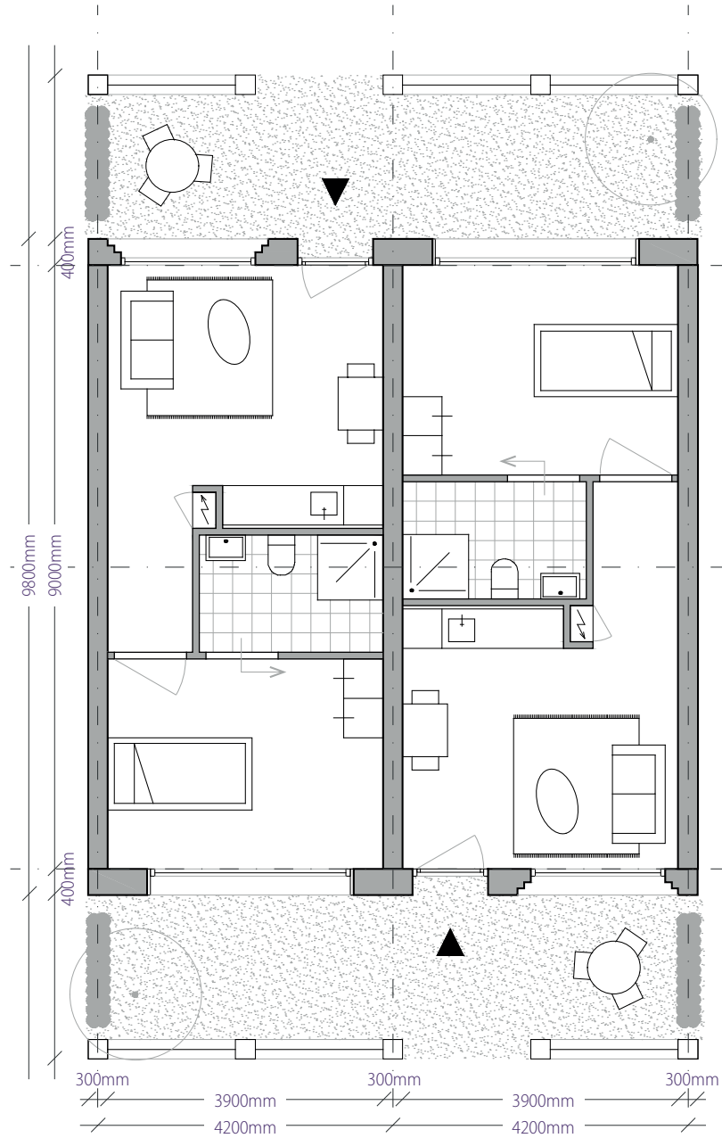
plattgrond type A 1:100
