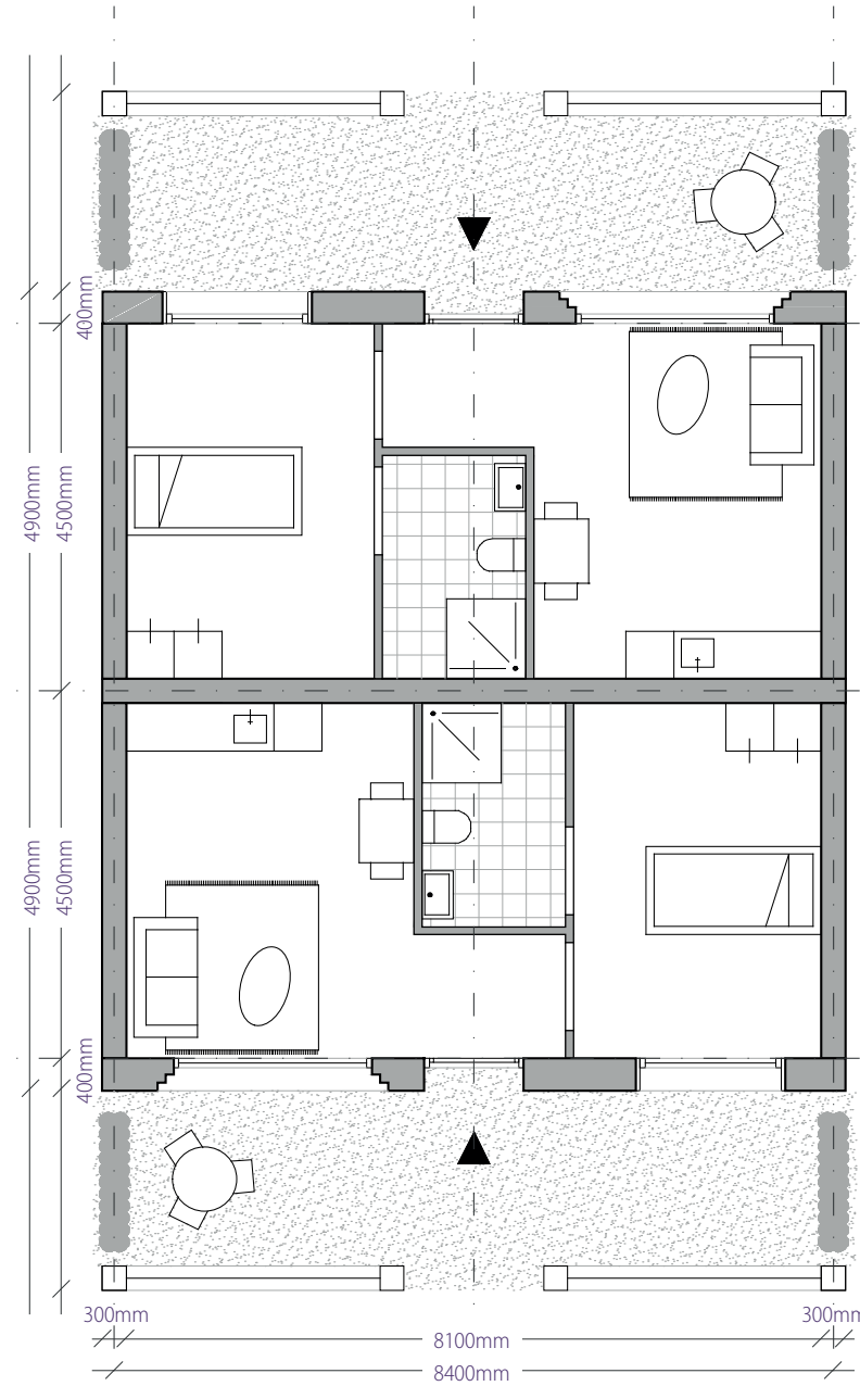
plattgrond type B 1:100
