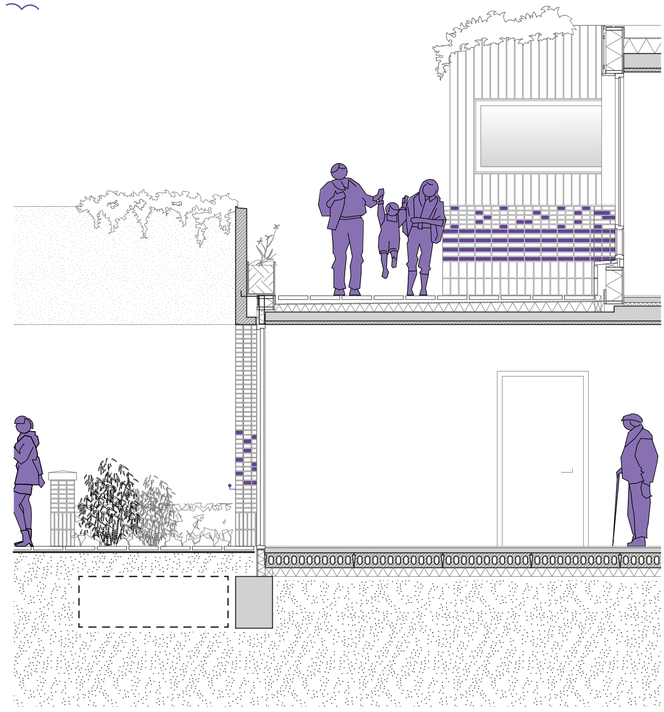
fragmentdoorsnede 1: 50
