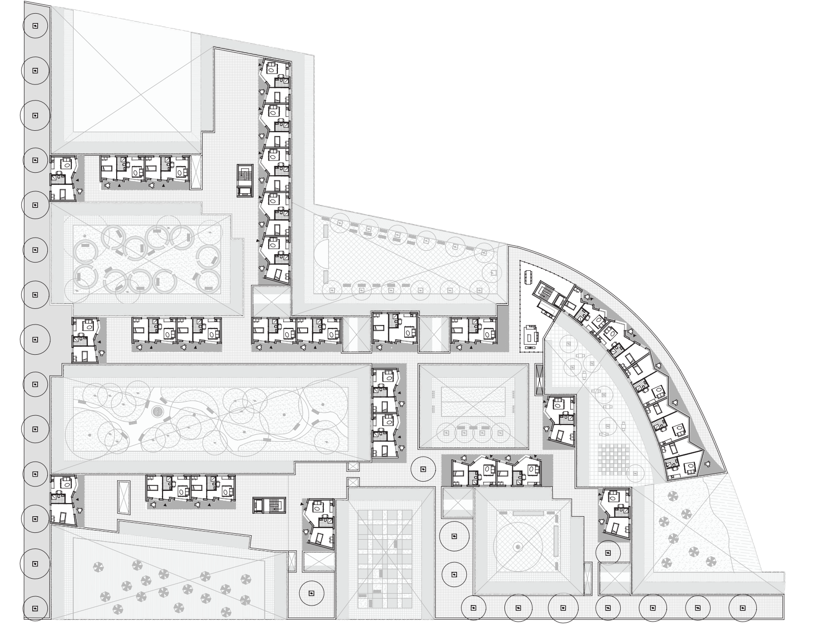
eerste verdieping 1: 750
