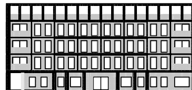
voor- en achteraanzicht 1:200
