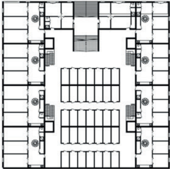
EERSTE VERDIEPING 1:200
