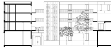
Doorsnede AA 120
