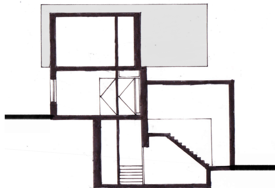
Dwars Doorsnede
