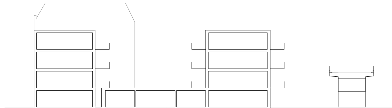
langsdoorsnede
