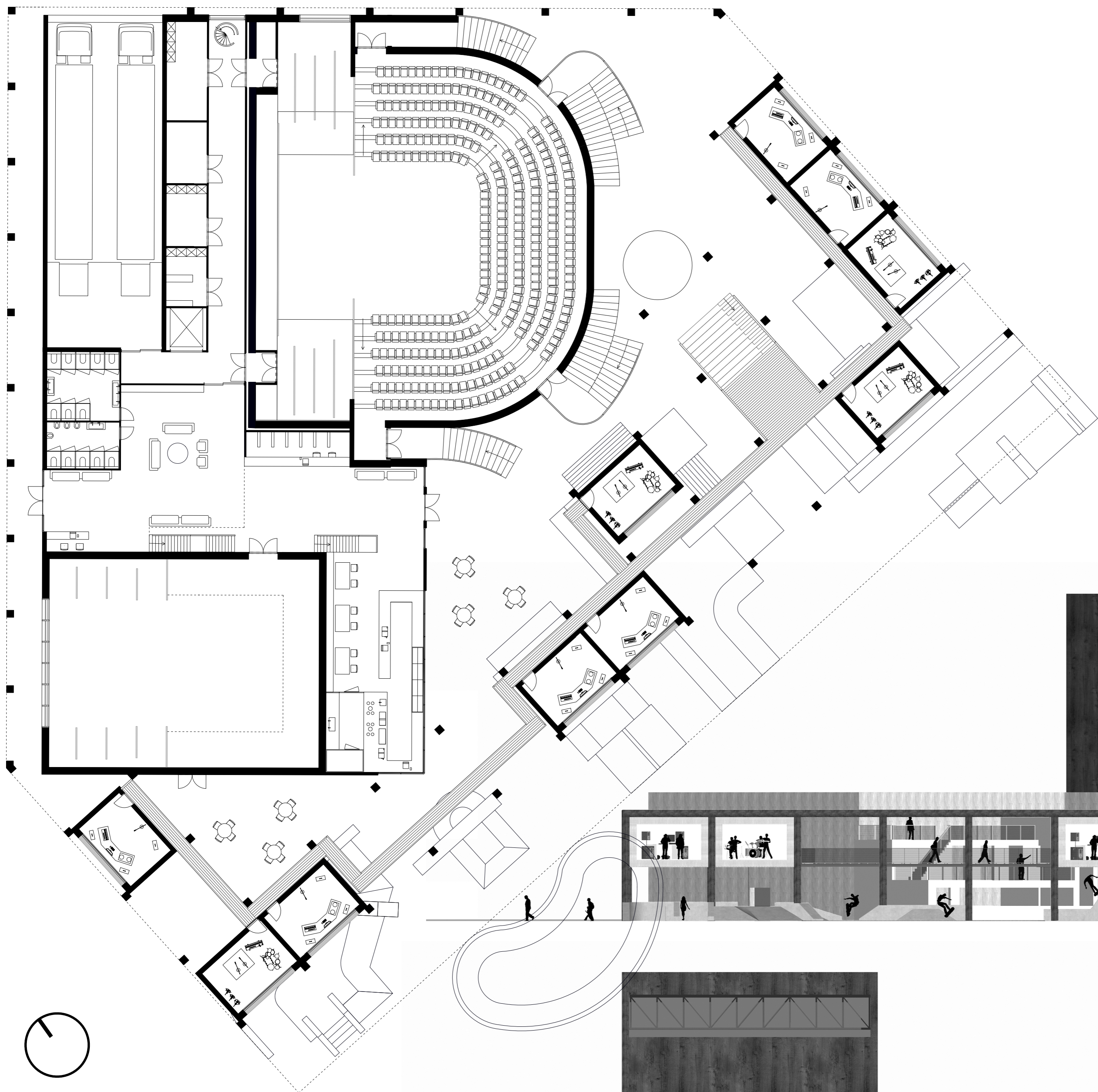
PLATTEGROND 1:200
