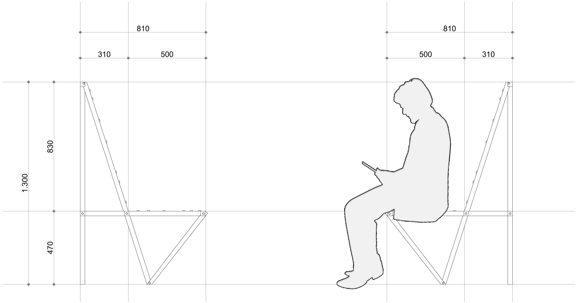
Doorsnede
