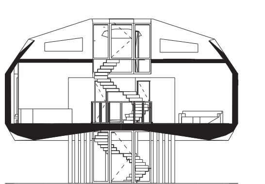
doorsnede AA
