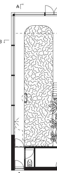
begane grond
