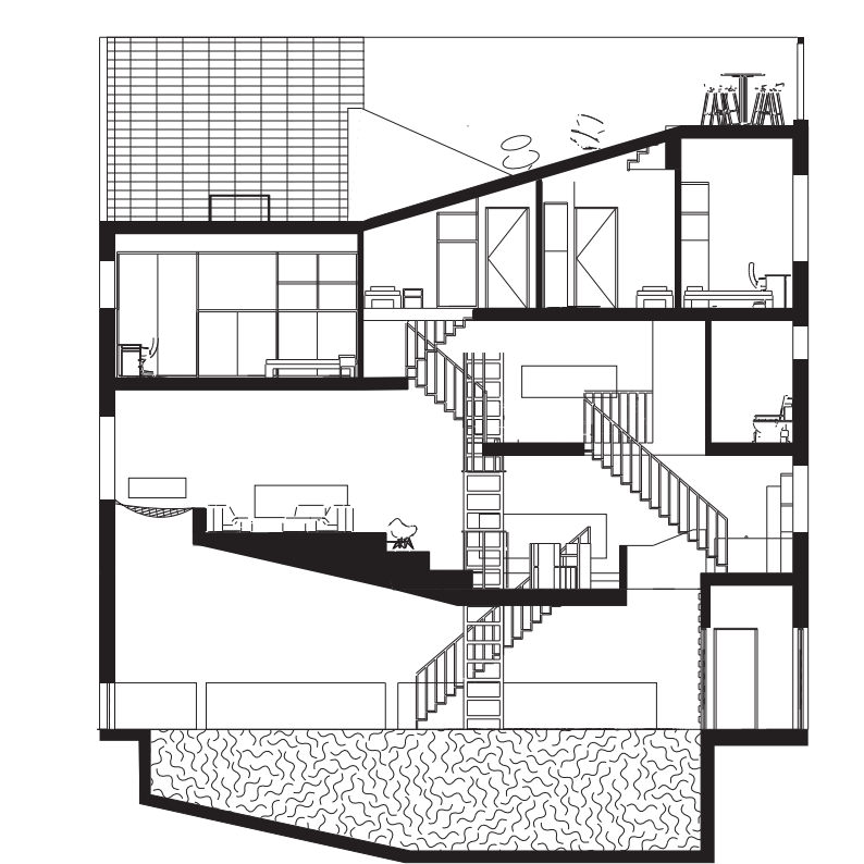
doorsnede AA
