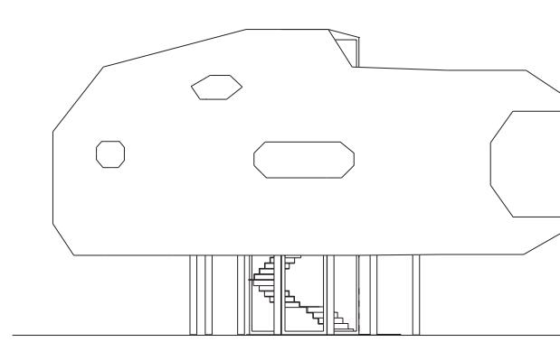
aanzicht zuid
