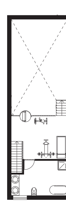
teende verdieping
