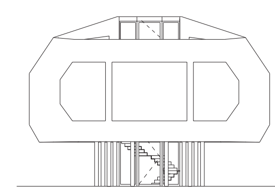
aanzicht west
