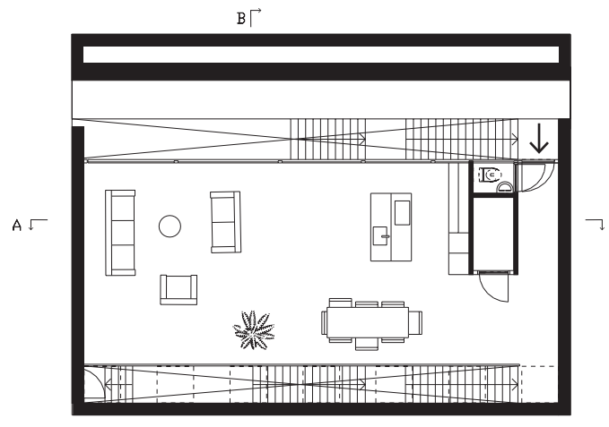
begane grond
