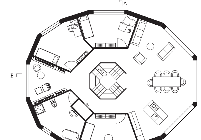
eerste verdieping
