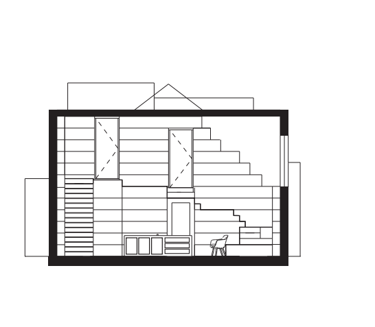
doorsnede BB
