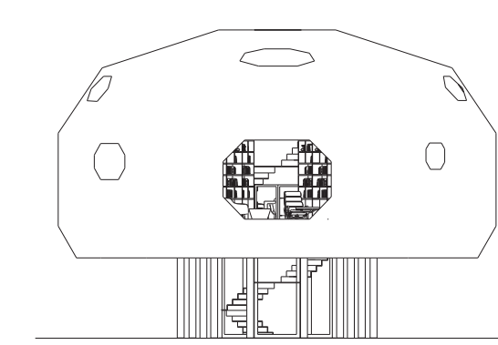
aanzicht oost
