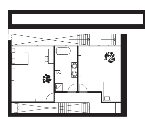
eerste verdieping
