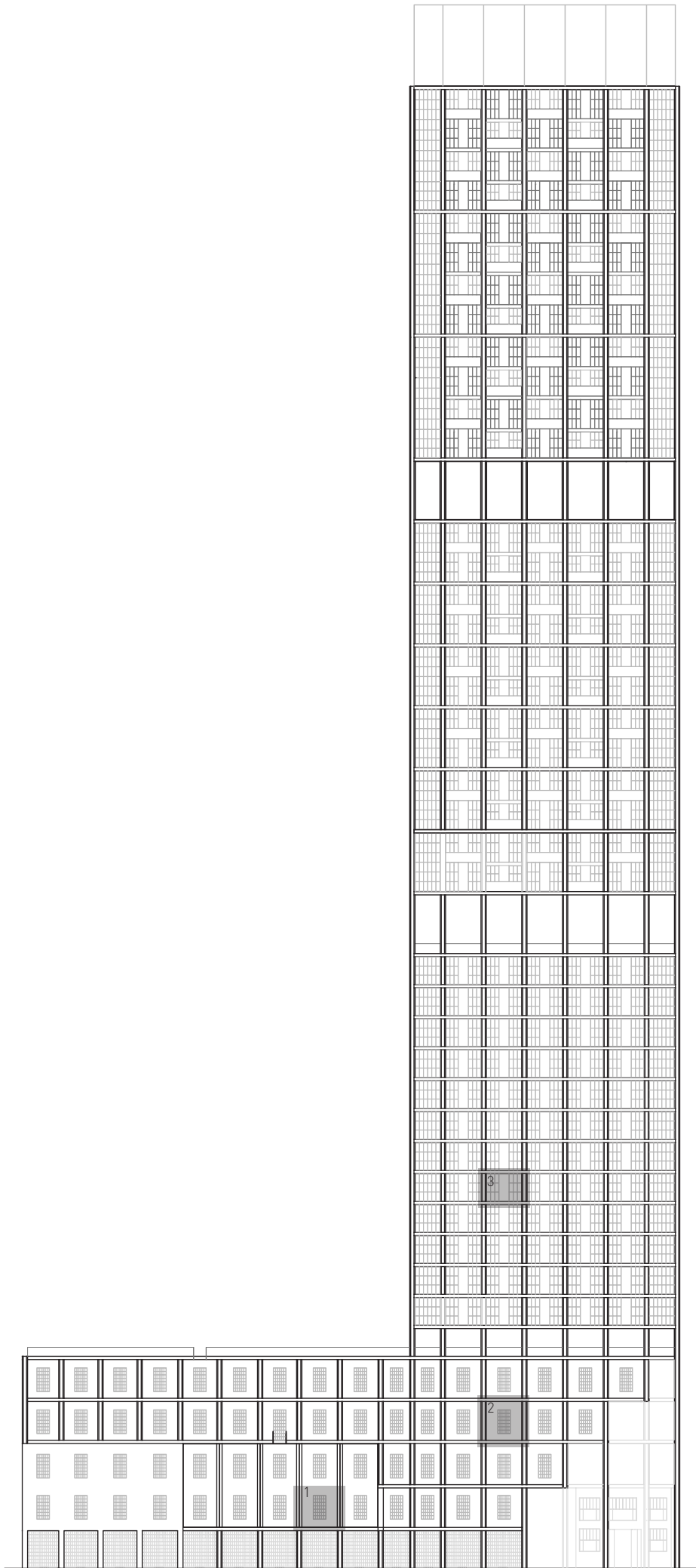
Gevelaanzicht Noord-Oost
