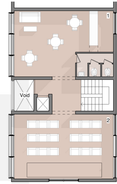
2DE VERDIEPING
