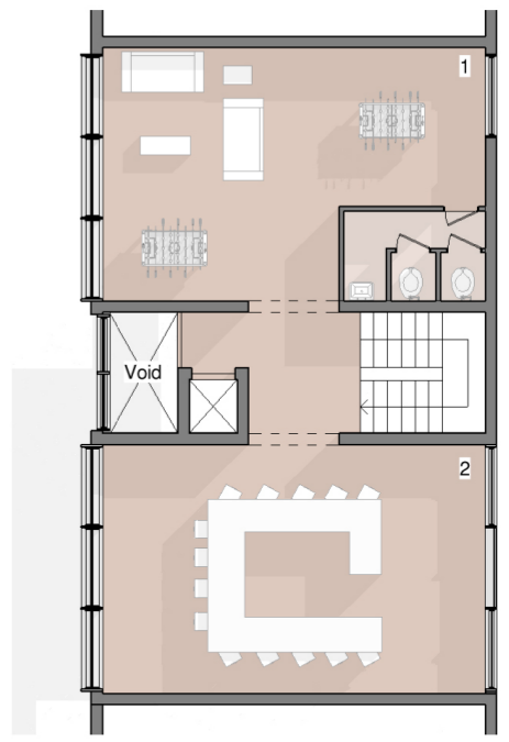
2 DE VERDIEPING
