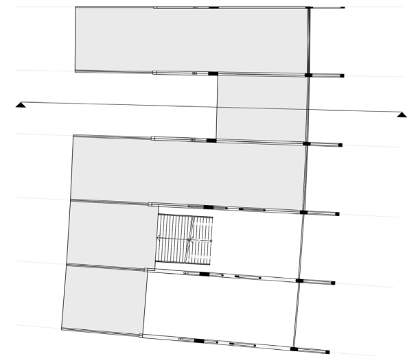
Tweede verdieping 1:200
