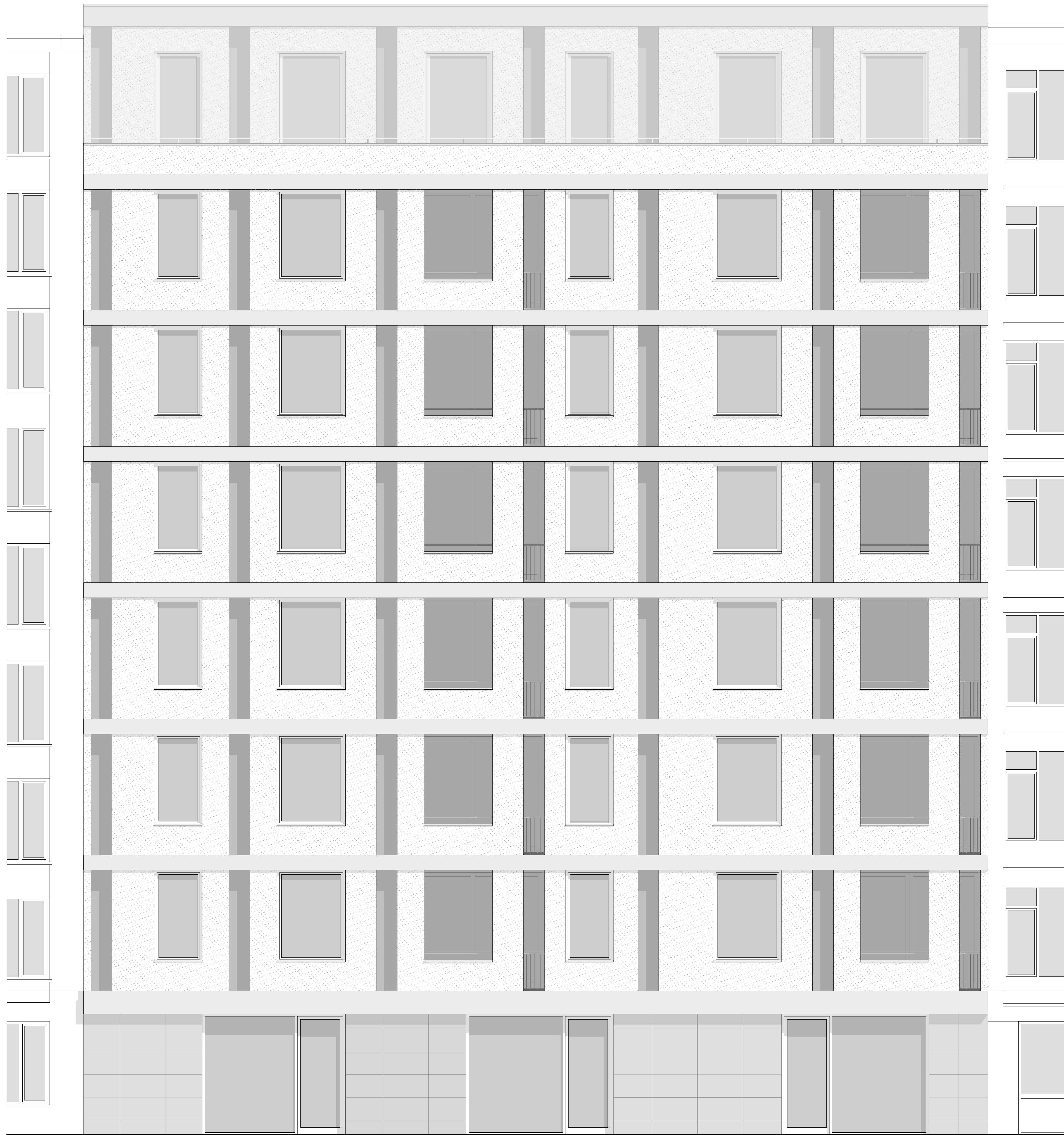
Gewestricht 1:50
