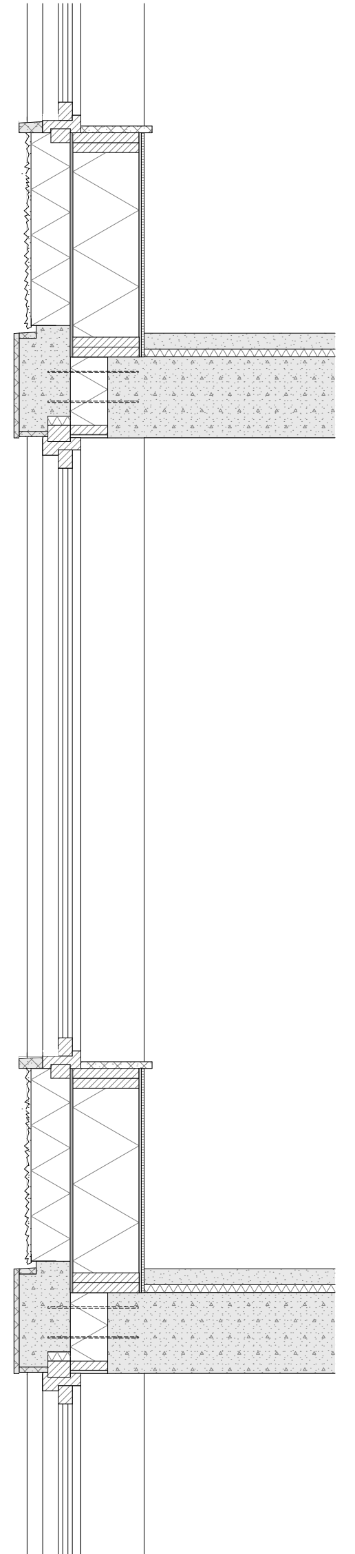
Doorsnede 1:20
