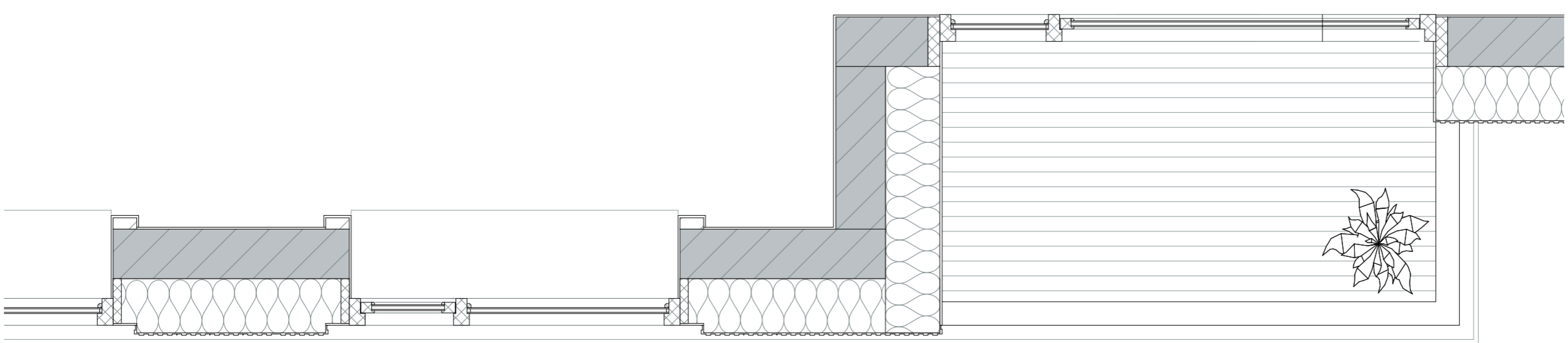
horizontale snede 1:20
