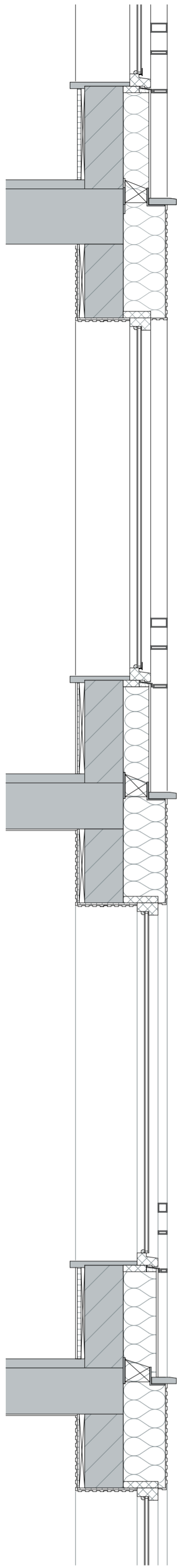
verticale snede 1:20
