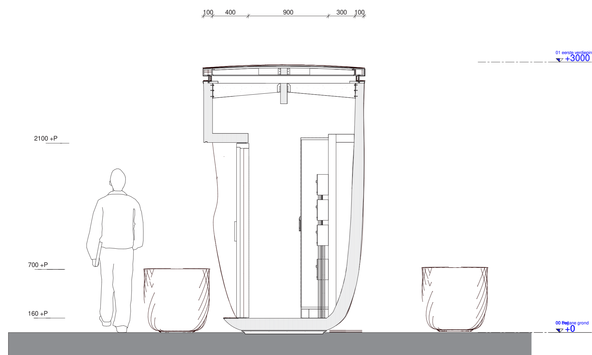
Doorsnede gebouw - 1:20
