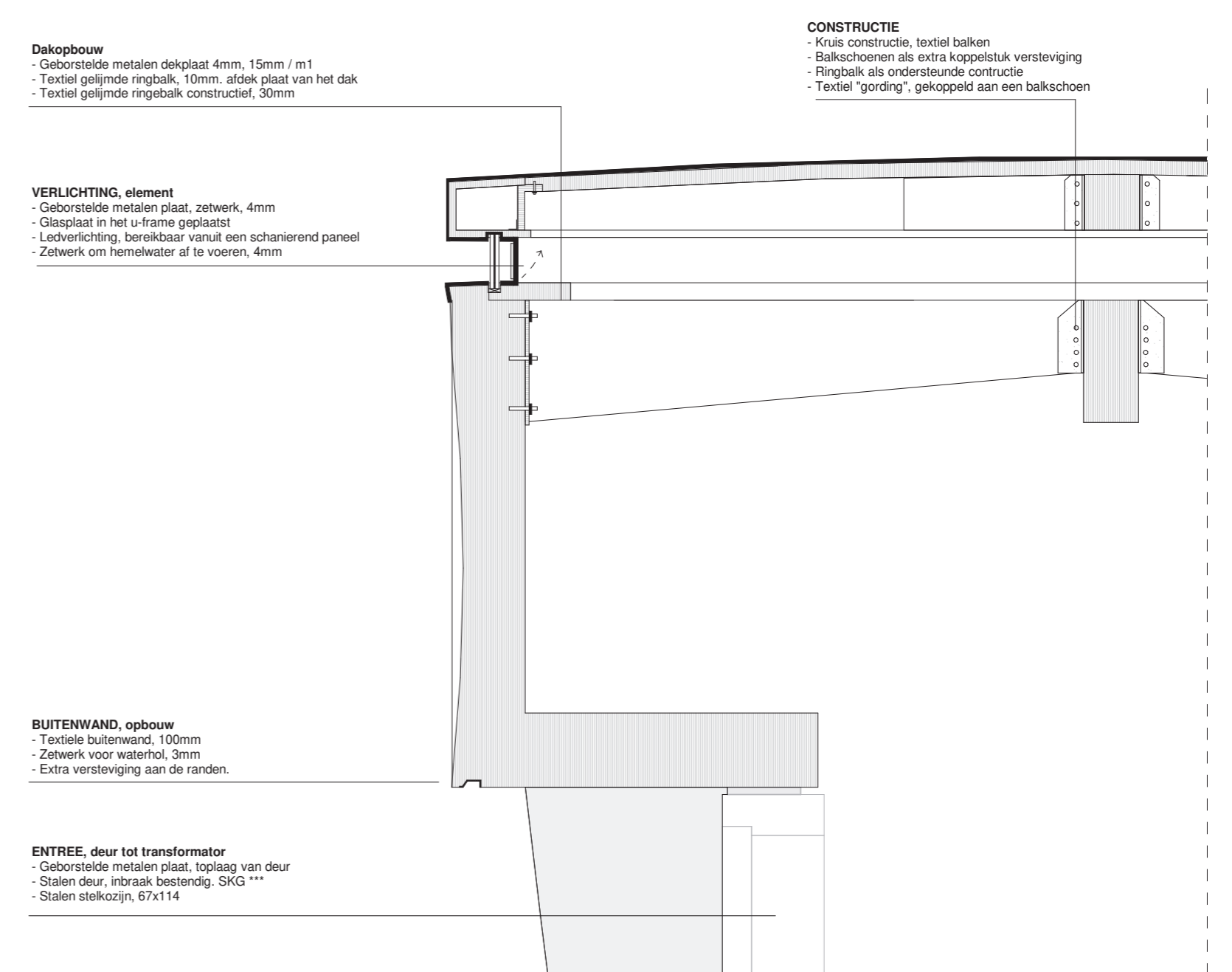
Principe detail, dak aansluiting - 1:5
