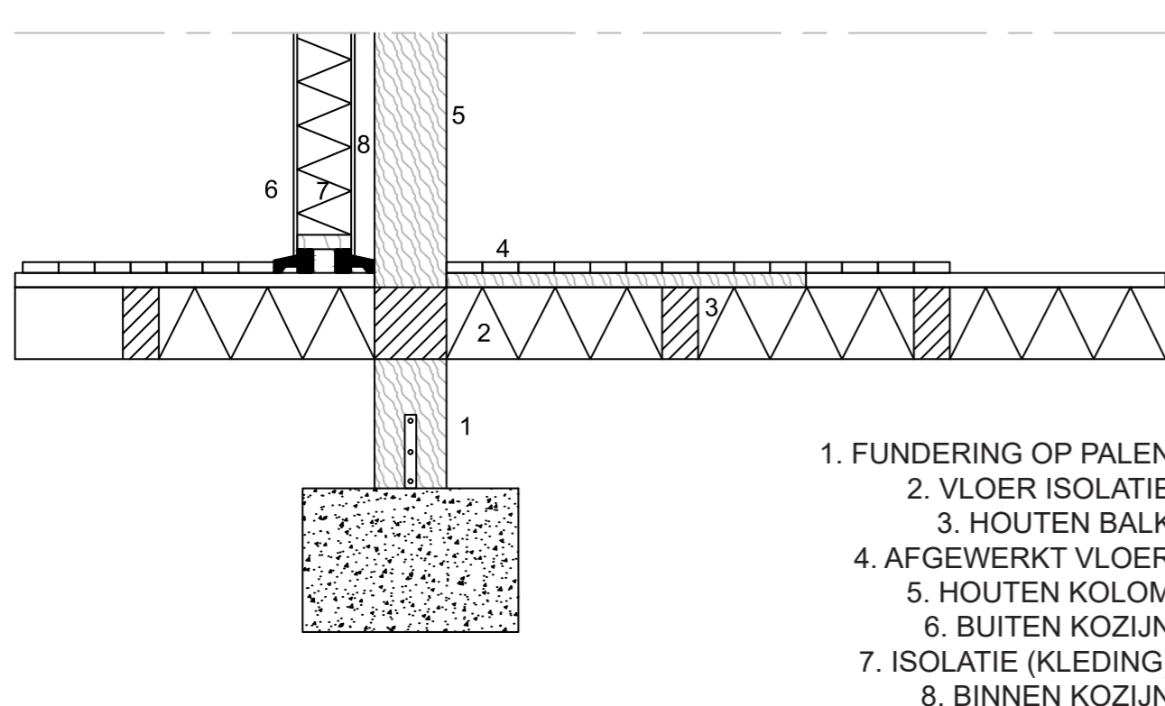
AANSLUITING RAAMKOZIJN OP VLOER
