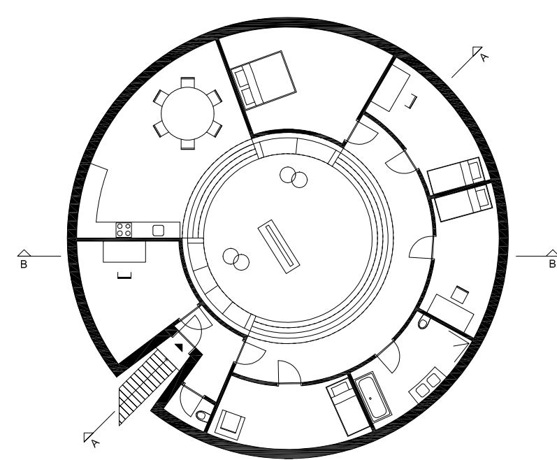
eerste verdieping
