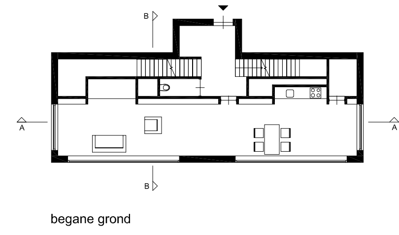
begane grond
