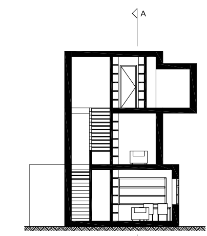
doorsnede B-B
