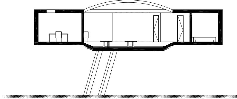
doorsnede B-B
