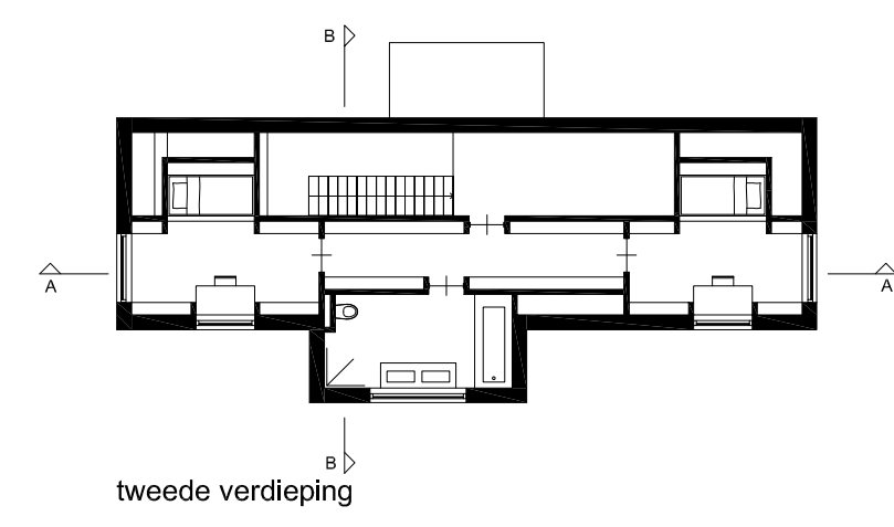
tweede verdieping
