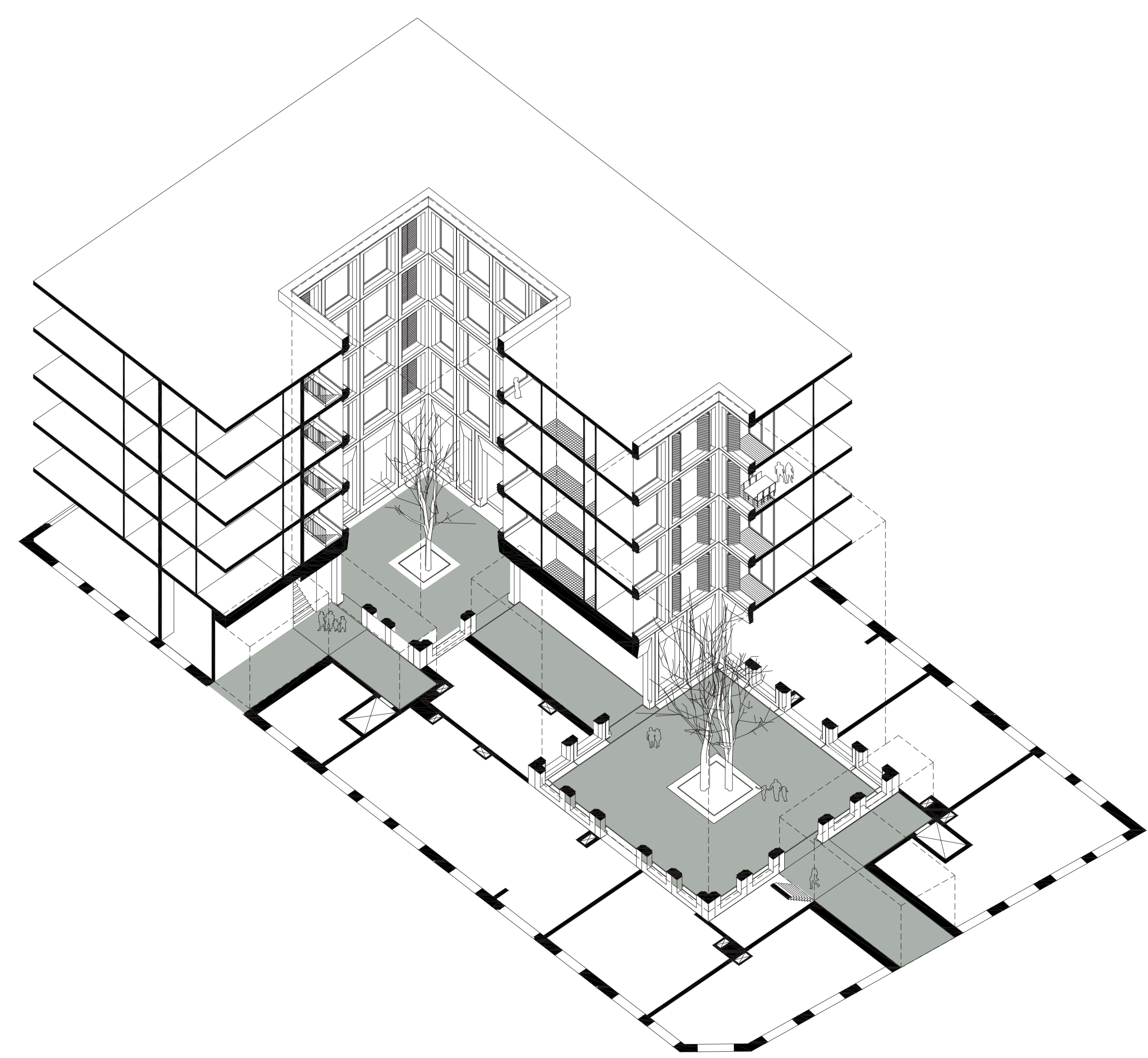
axonomerie | 1:200
