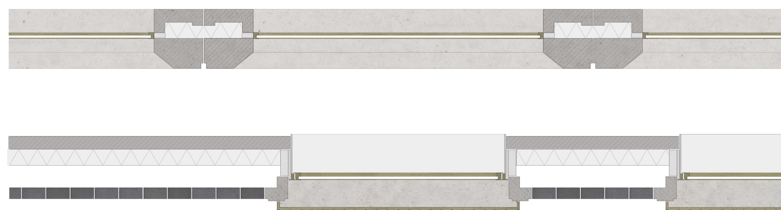
GEVEL 'VIA DELLA CONCILIAZIONE' FRAGMENT 1:20
