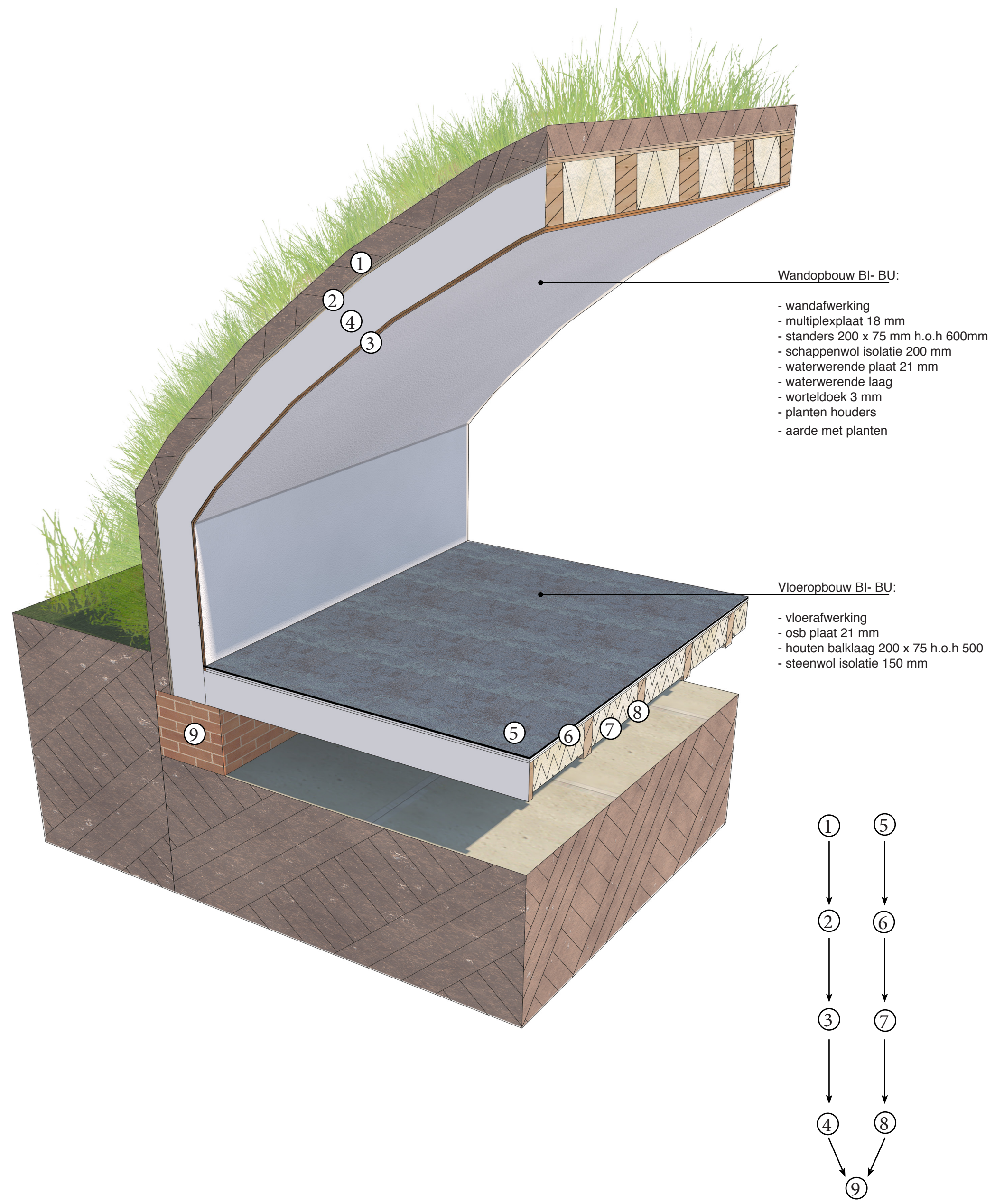
Demontage volgorde
