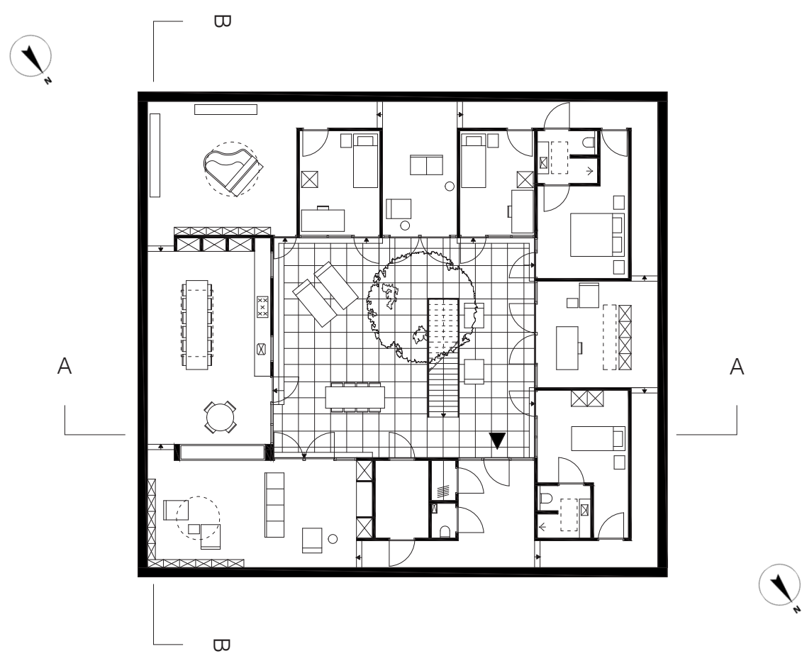
Begane grond
