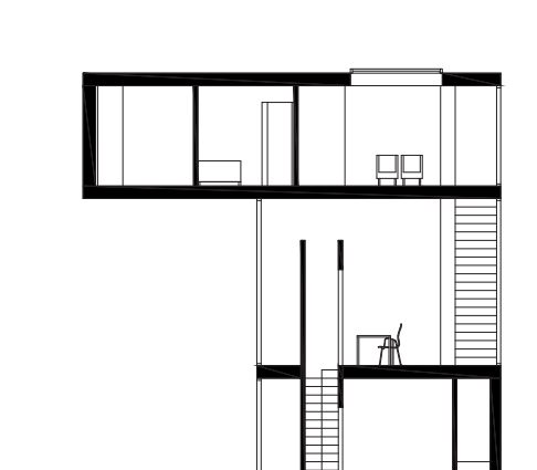
Doorsnede B
