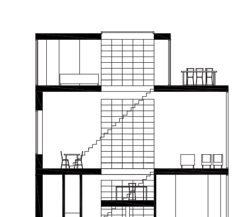
Doorsnede A
