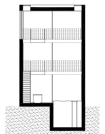
Doorsnede B
