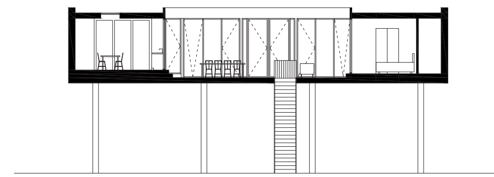
Doorsnede A
