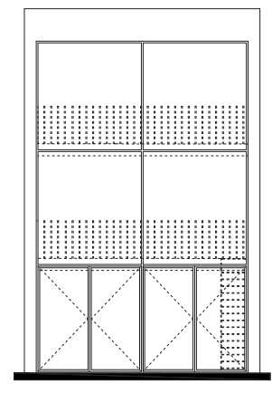
Gevel zuid
