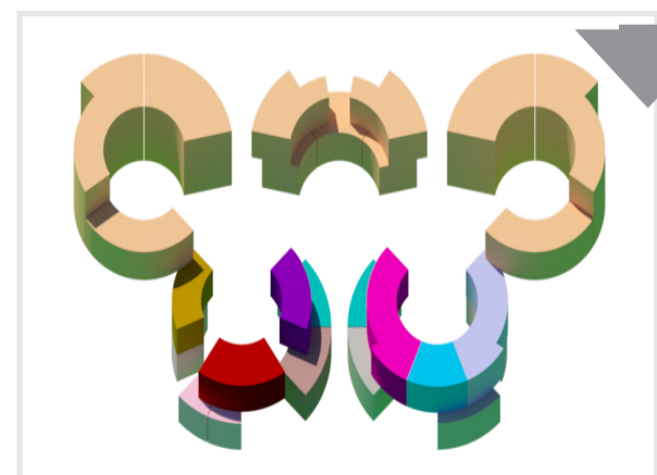
Diagram 3, Functies
