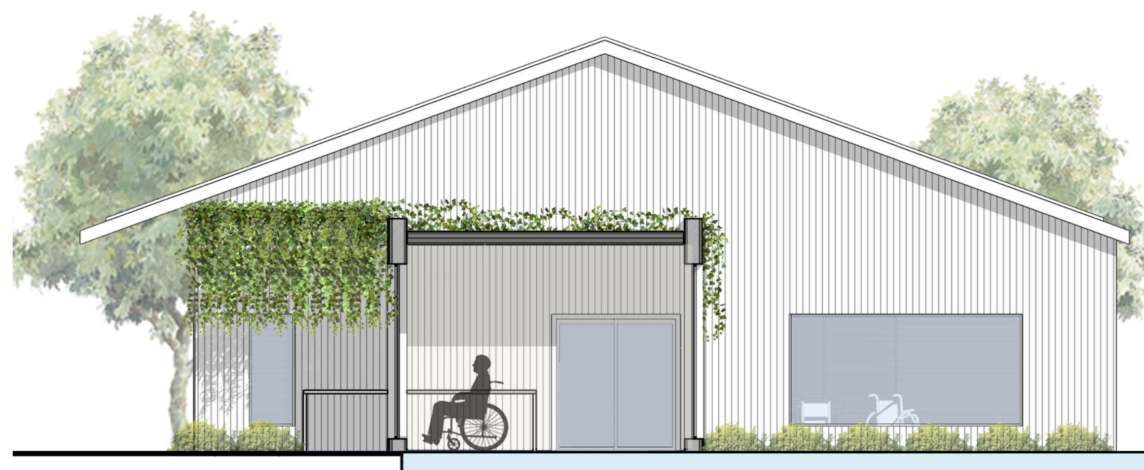
D: PRINCIPE DOORSNEDE SC: 1.100
