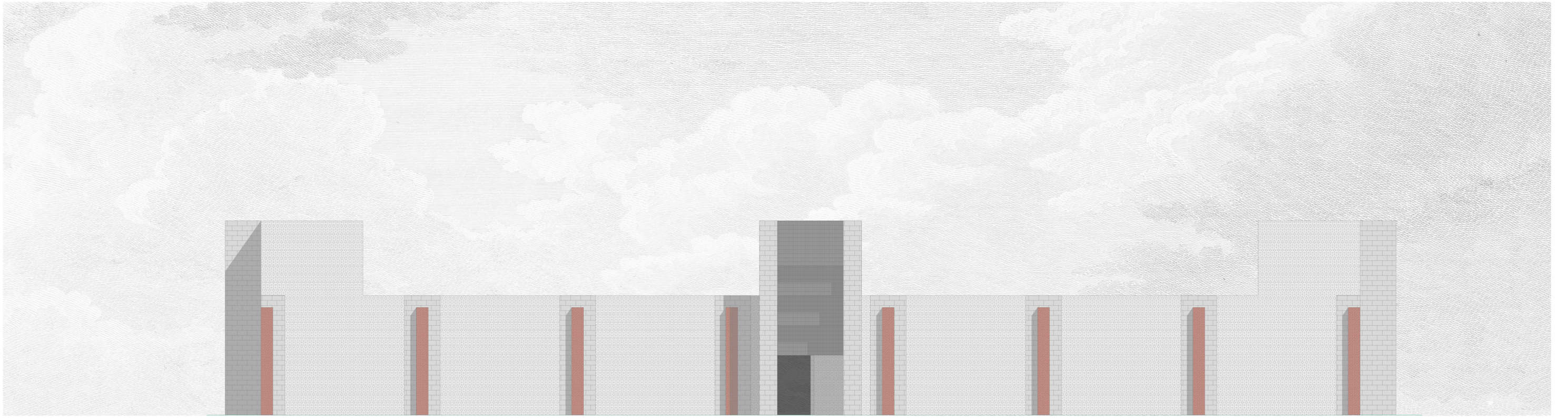
Gevelaanzicht crypte 1:200
