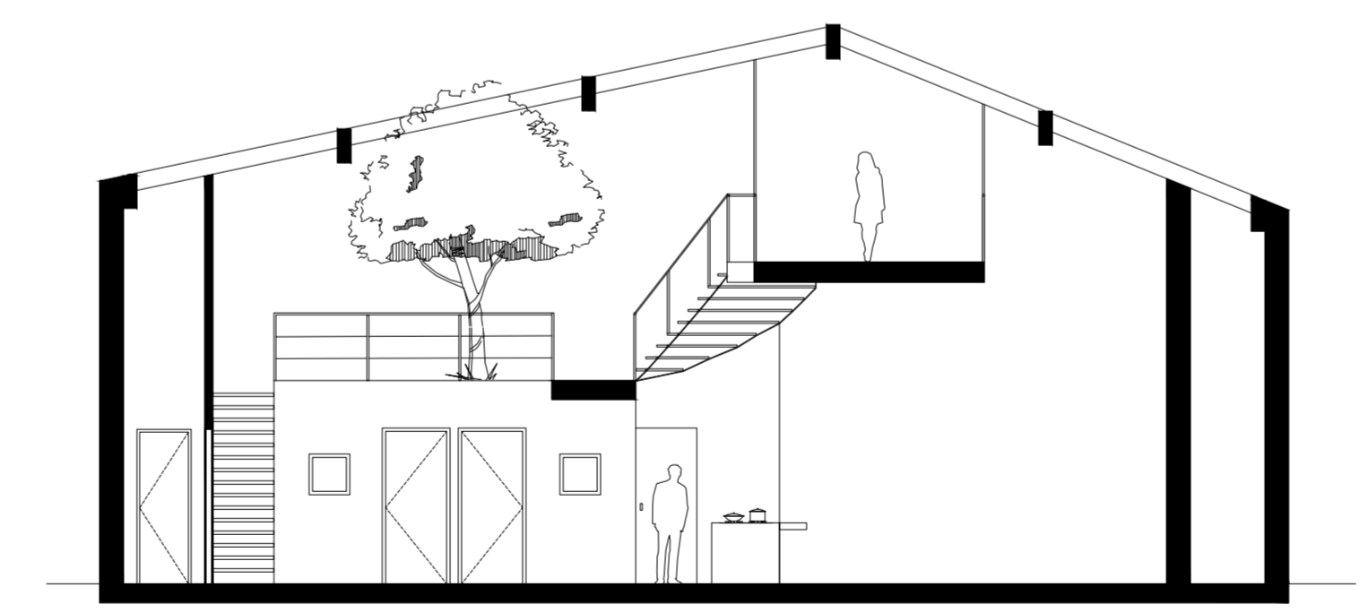
Doorsnede A
