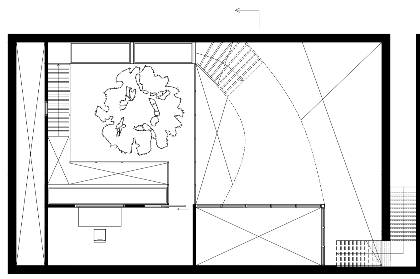
Eerste verdieping
