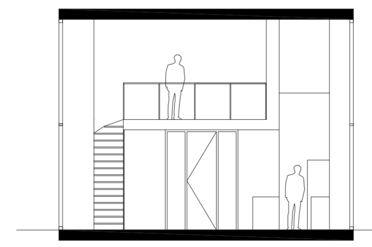
Doorsnede B
