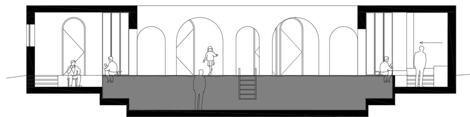
Doorsnede A
