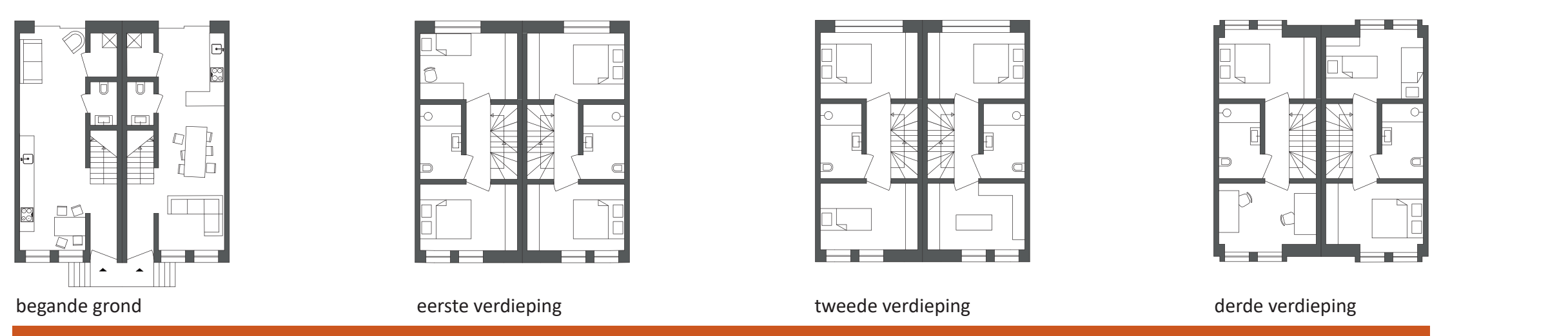
Type B rijtjeswoning
