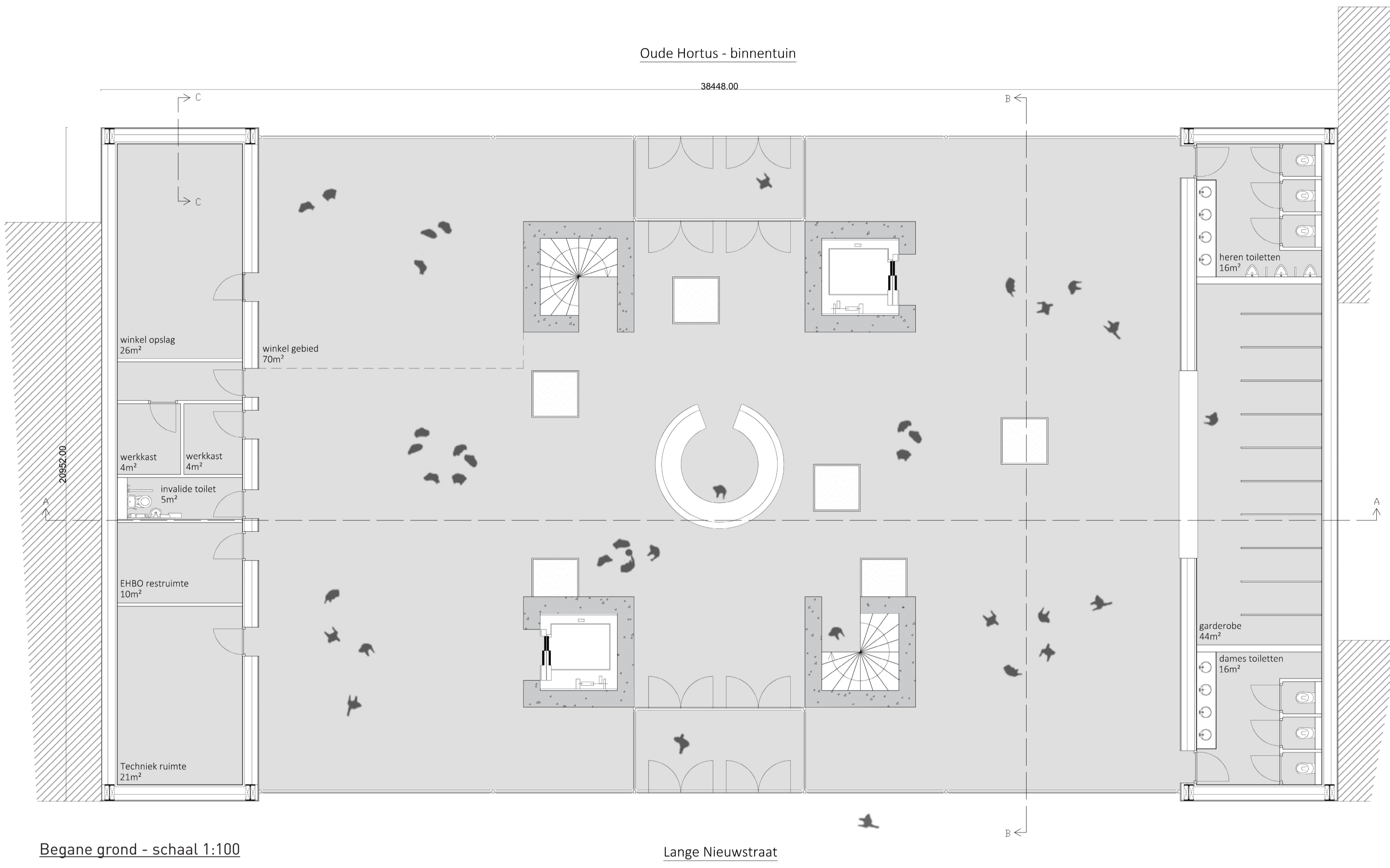
Begane grond - schaal 1:100
