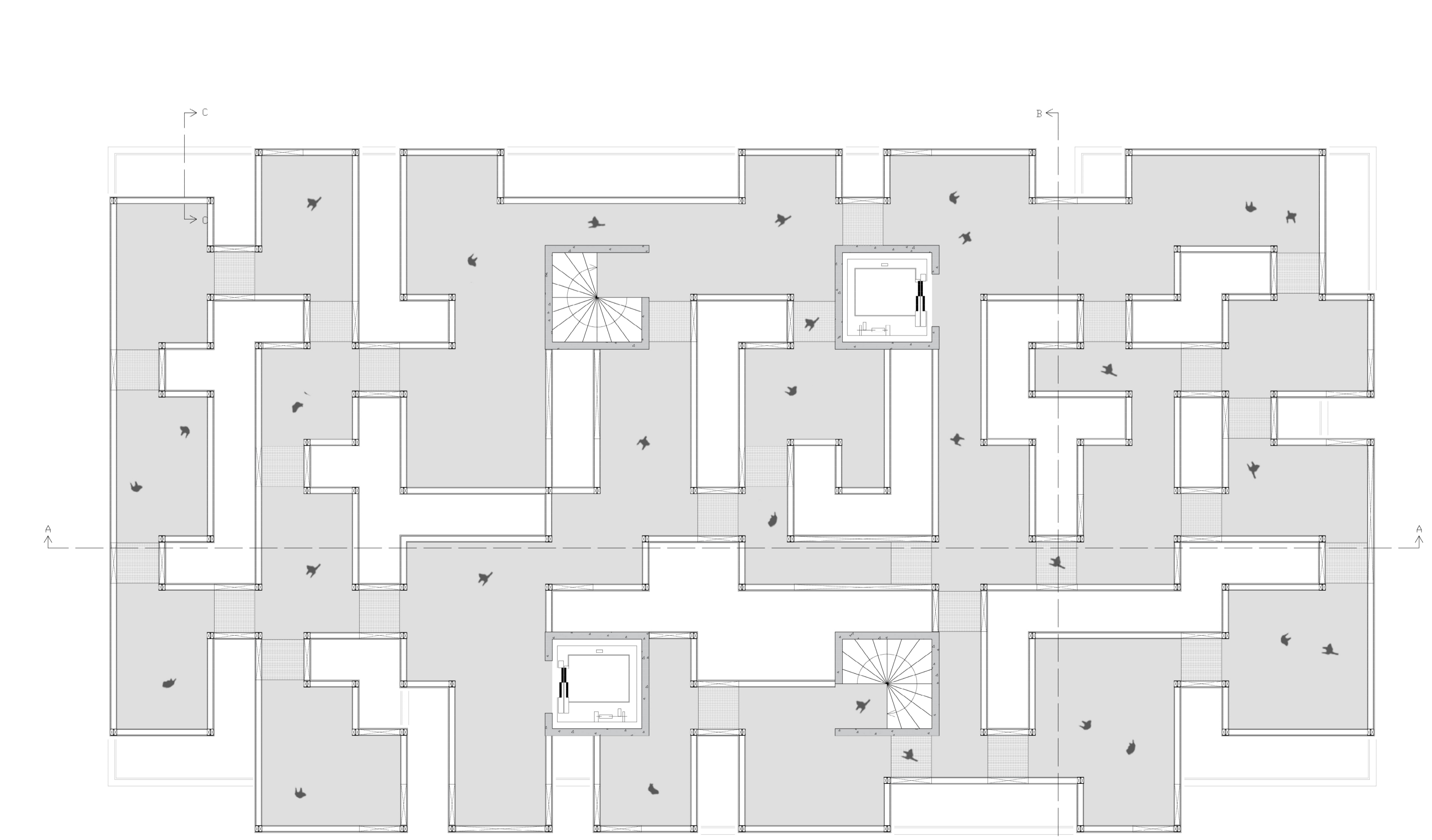
derde verdieping - schaal 1:100
