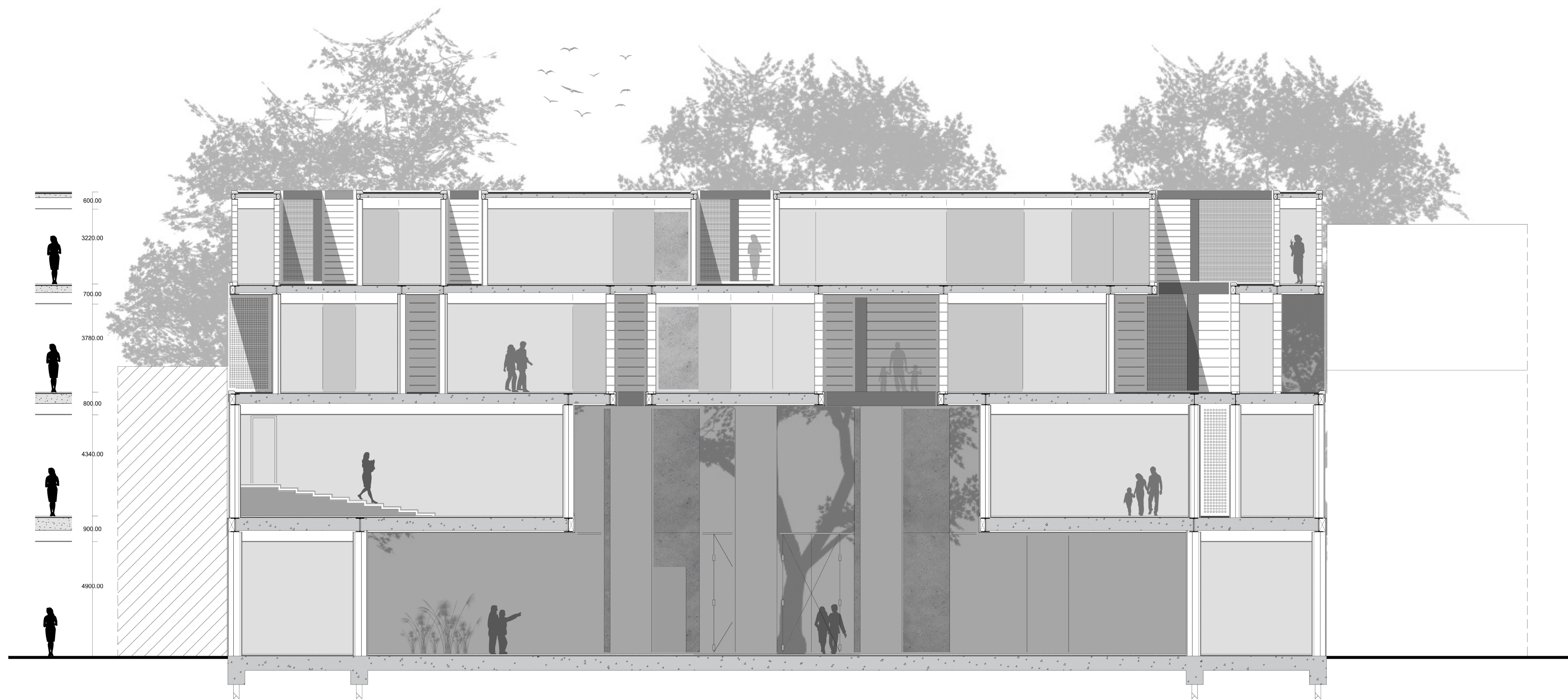
Doorsnede A - schaal 1:100
