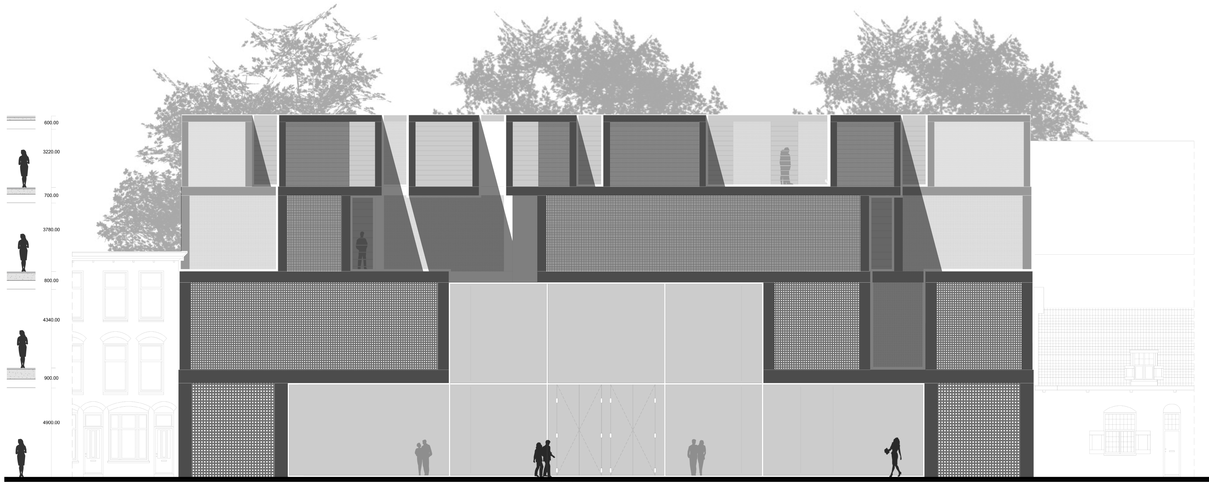
Voorgevel - schaal 1:100
