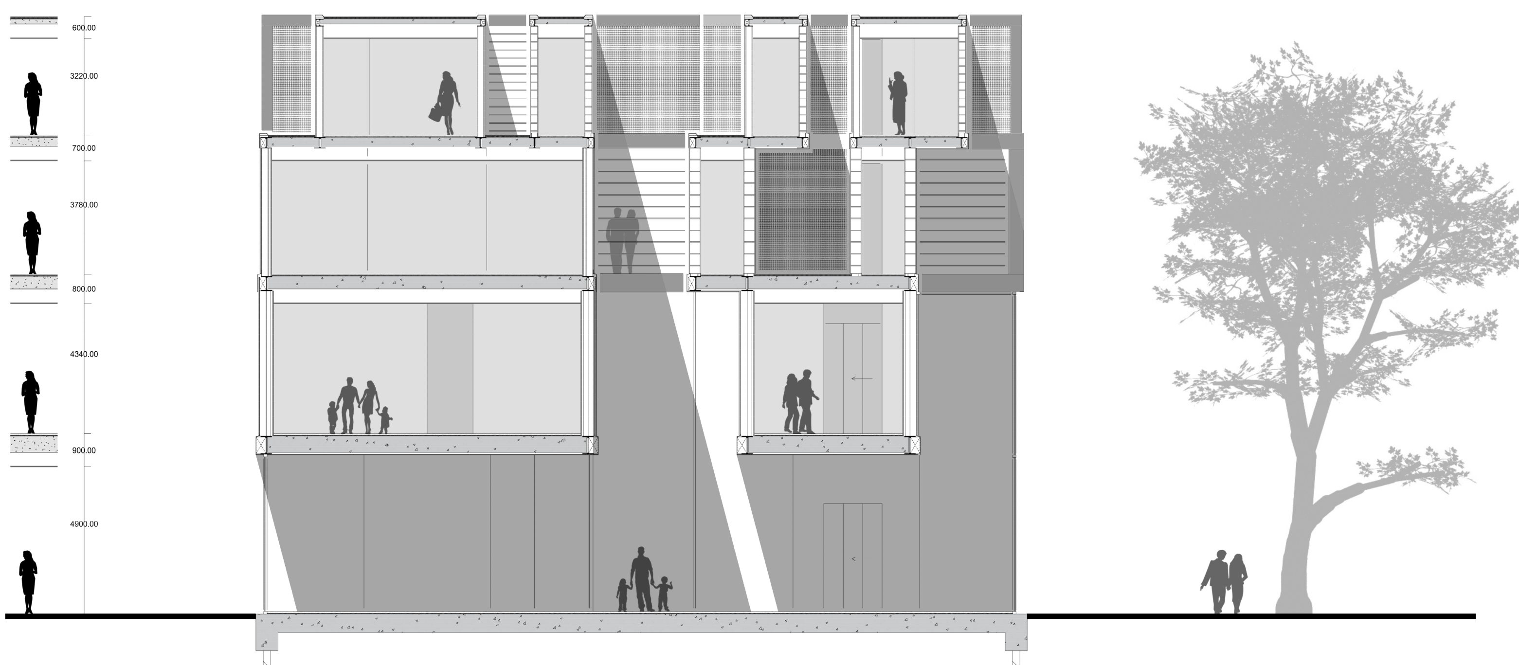
Doorsnede B - schaal 1:100
