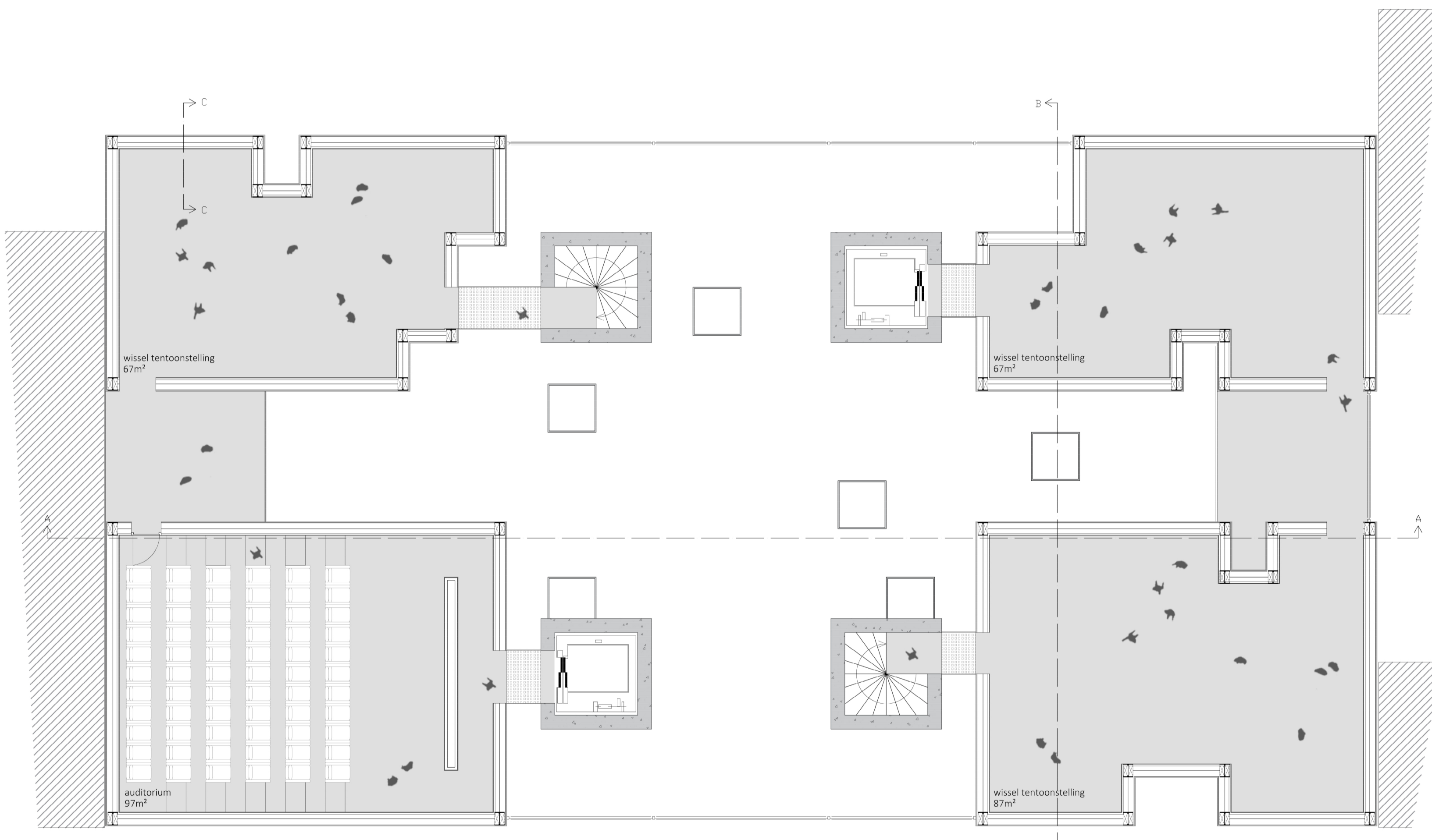
eerste verdieping - schaal 1:100
