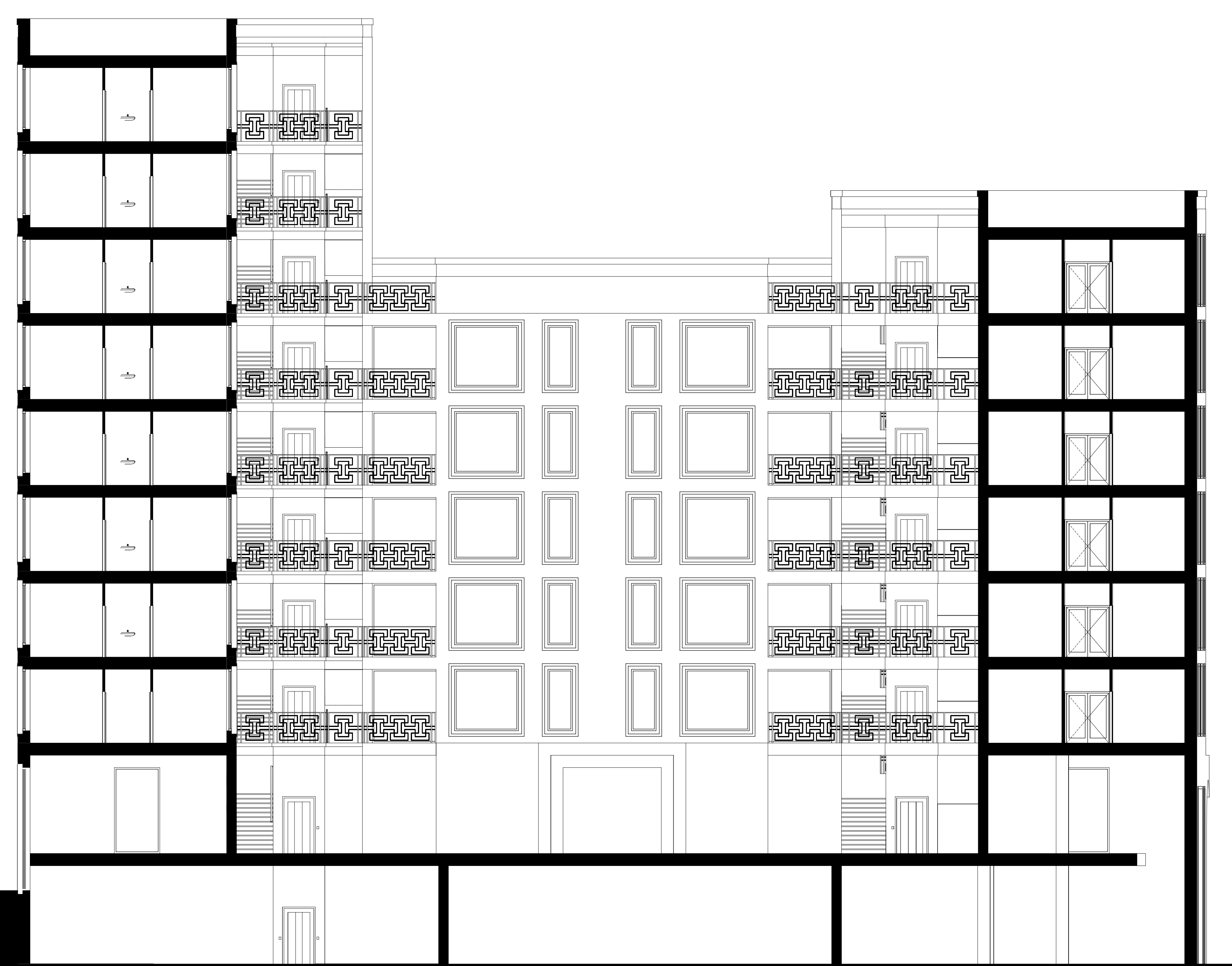
Longitudinal | 1:100
