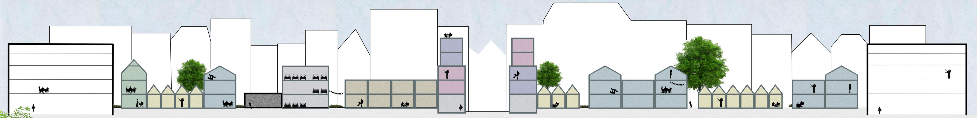
Een geboren woonstraat voor de nieuwe Amsterdamer, een feestje om in te wonen - langdoorsnede
