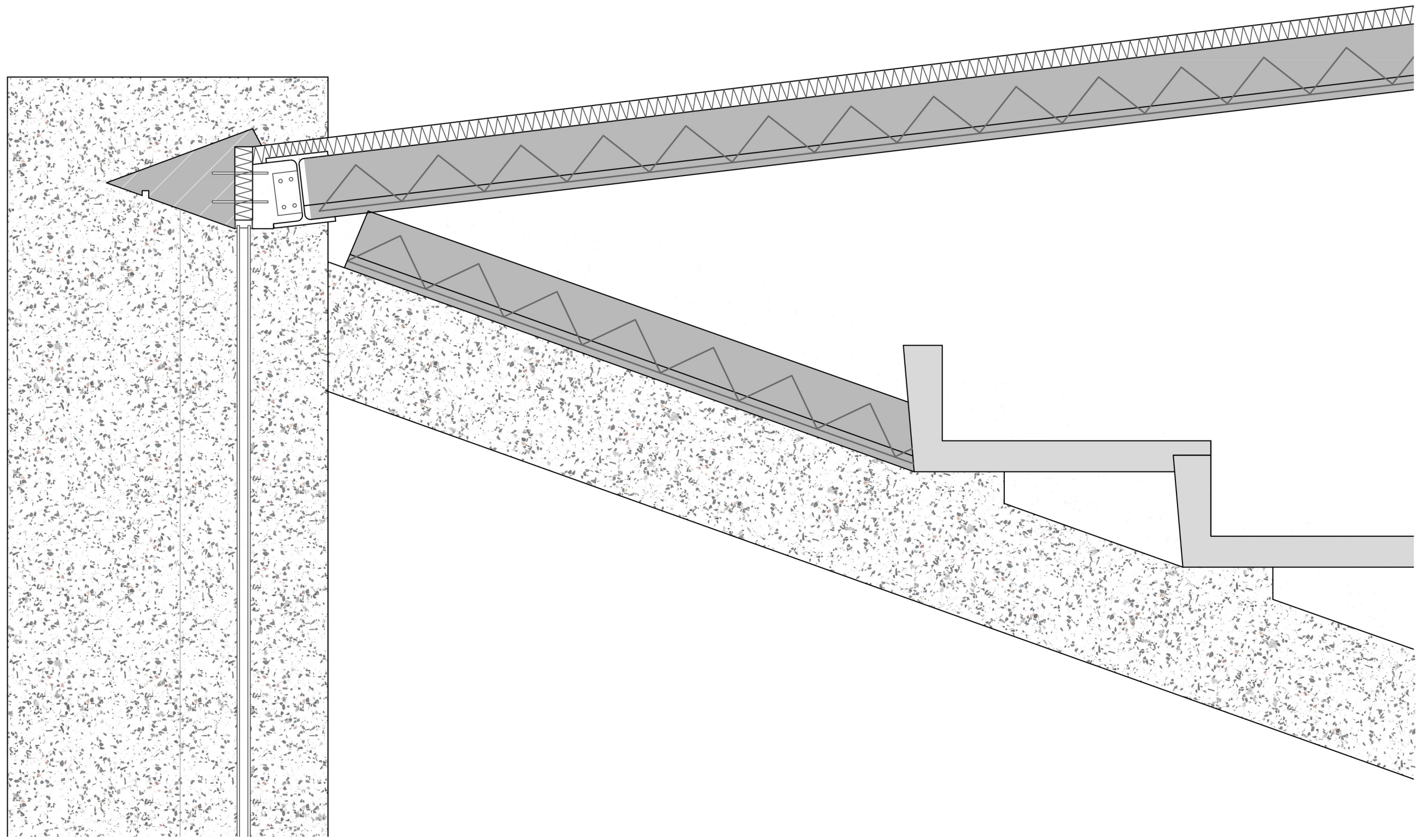
Fragment 1:20
