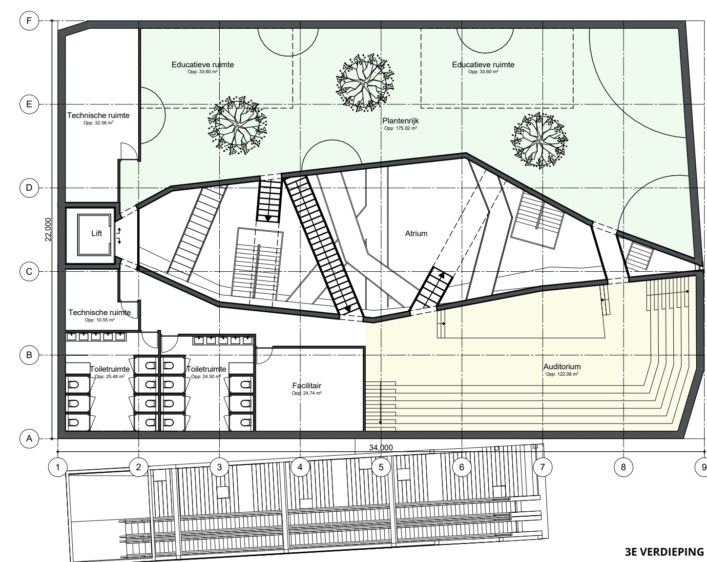
3E VERDIEPING 13500 m²
