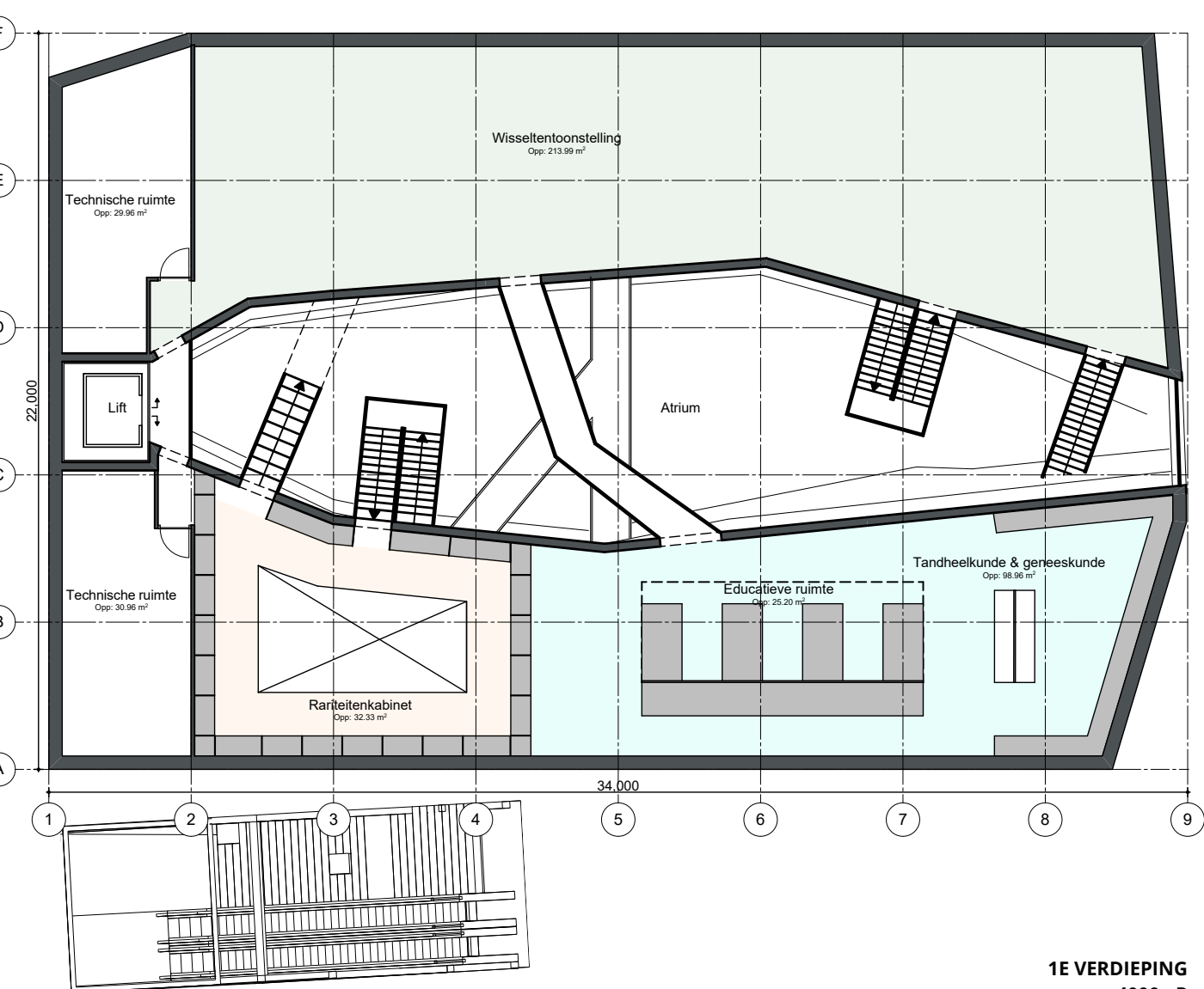
1E VERDIEPING 4000 m²
