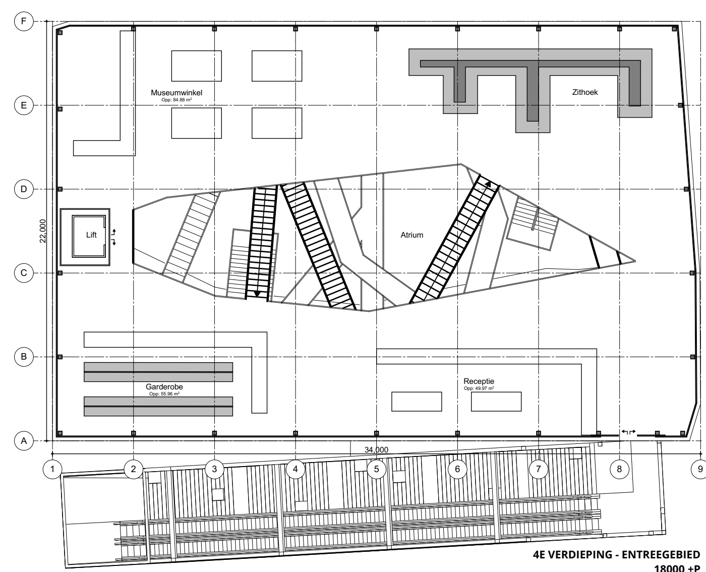
4E VERDIEPING - ENTREEGEBIED 18000 m²
