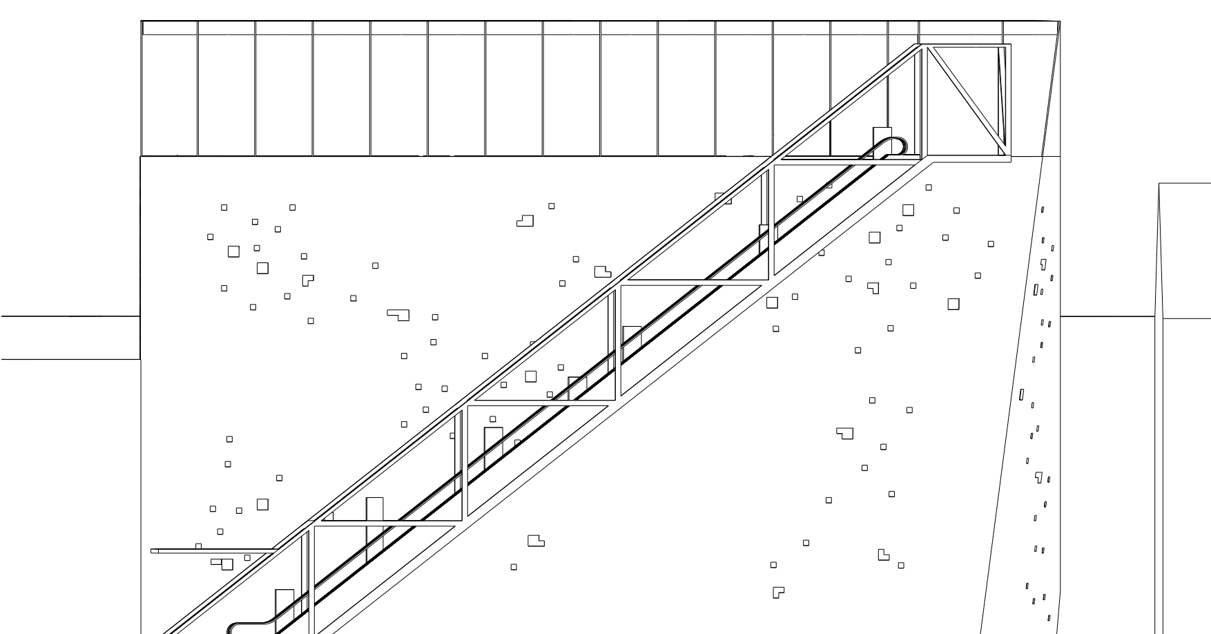
VOORGEVEL - LANGE NIEUWSTRAAT
