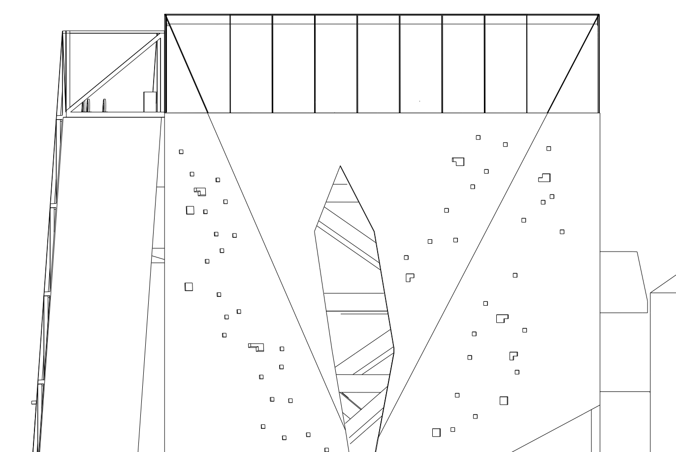
RECHTERZIJGEVEL
