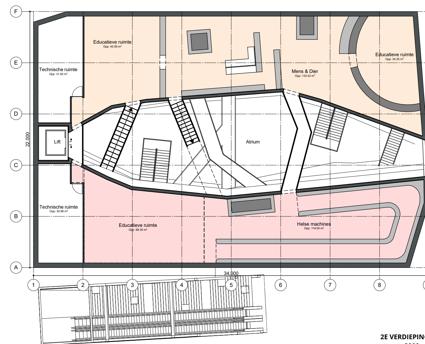
2E VERDIEPING 8000 m²
