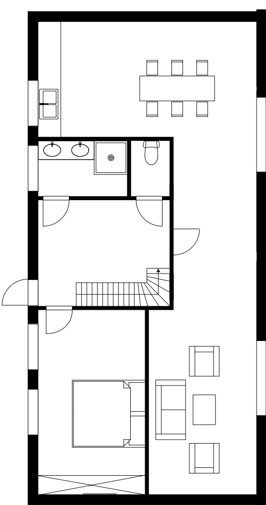
100 M² 1:1000
